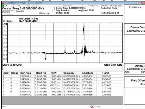
Band77-Part27 60MHz CP OFDM SCS30kHz QPSK RB1 161 Chain0 CH633334
