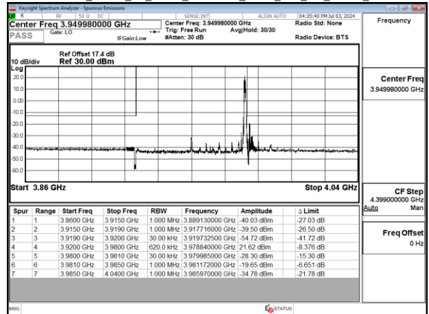
Band77-Part27 60MHz CP OFDM SCS30kHz QPSK RB1 161 Chain0 CH663332
