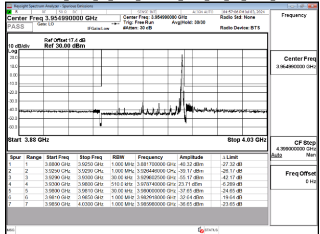
Band77-Part27_50MHz_CP_OFDM_SCS30kHz_QPSK_RB1_132_Chain0_CH663666
