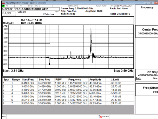
Band77-Part27 60MHz CP OFDM SCS30kHz QPSK RB1 161 Chain0 CH634666
