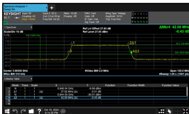
Figure 87 - 802.11ax HE40 SU LPI Minimum 99% OBW
