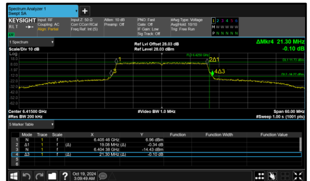
Figure 142 - 802.11ax HE20 SU SP Maximum 99% OBW
