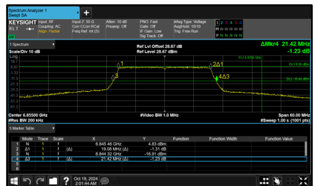
Figure 94 - 802.11ax HE20 SU SP Maximum 99% OBW
