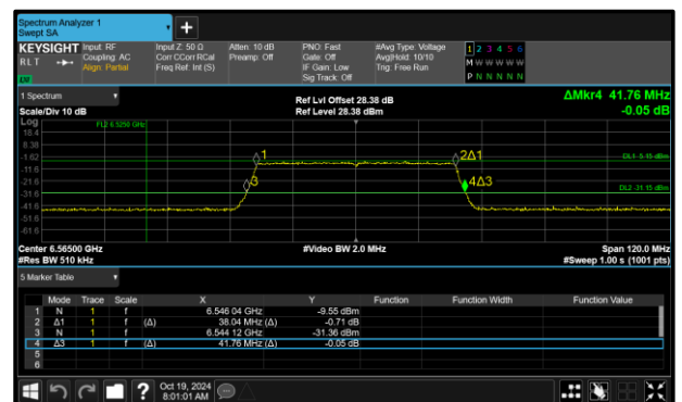
Figure 152 - 802.11ax HE40 SU VLP Maximum 99% OBW
