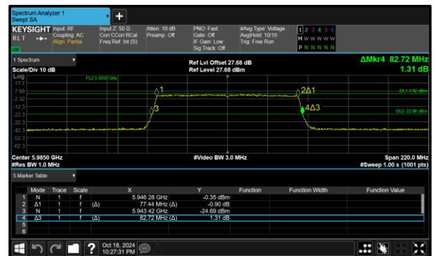
Figure 138 - 802.11ax HE80 SU LPI Maximum 99% OBW
