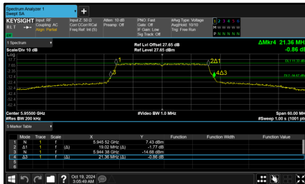
Figure 141 - 802.11ax HE20 SU SP Minimum 99% OBW
