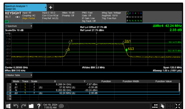
Figure 128 - 802.11ax HE40 SU VLP Maximum 26 dB EBW
