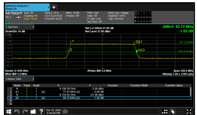
Figure 90 - 802.11ax HE80 SU LPI Maximum 99% OBW
