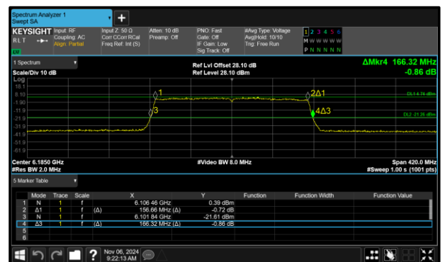
Figure 92 - 802.11ax HE160 SU LPI Maximum 99% OBW
