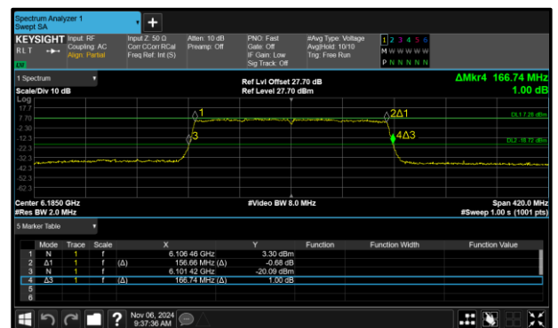
Figure 140 - 802.11ax HE160 SU LPI Maximum 99% OBW
