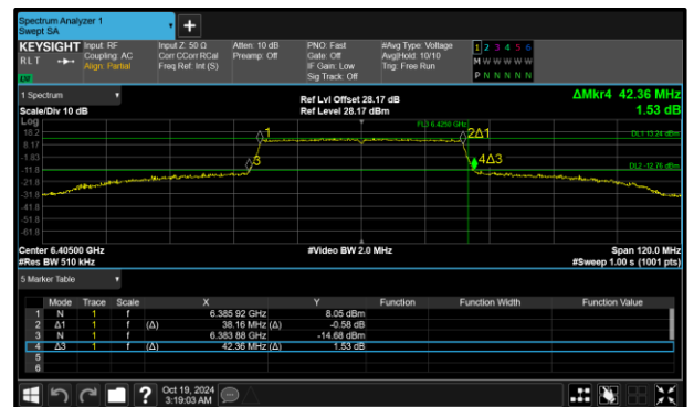
Figure 144 - 802.11ax HE40 SU SP Maximum 99% OBW
