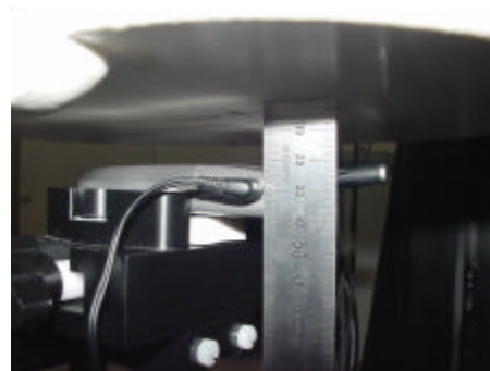
Fig. 22. Body SAR Test
