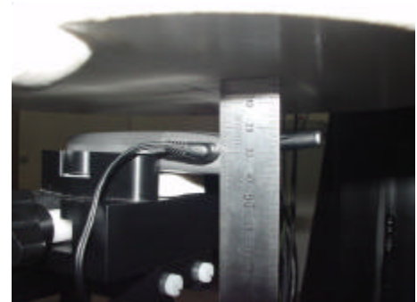
Fig. 21. Body SAR Test Setup
