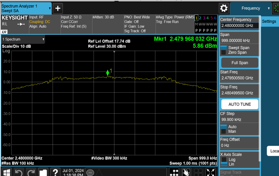
BLE 1M-Ant1-2480-PASS
