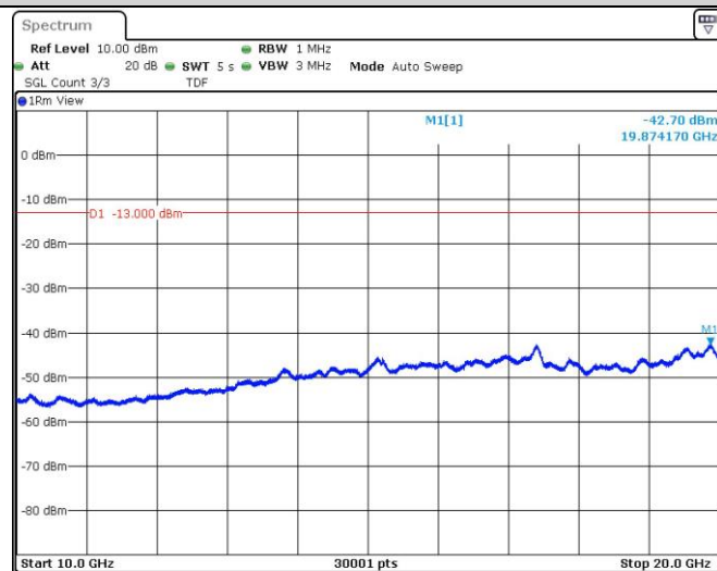
Band4-1413-2-10000~20000MHz
