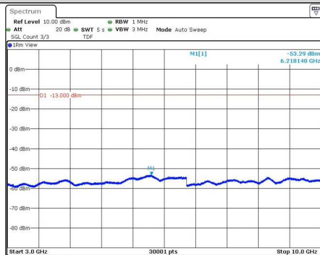
Band2-9538-3-3000~10000MHz
