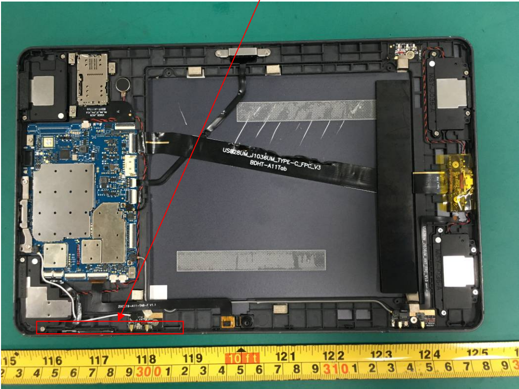
BT/WIFI/GPS Antenna
