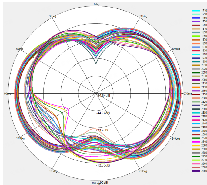
WCDMA B4/LTE B4/B7/B66 NR n7/n66 \Phi=90^\circ
