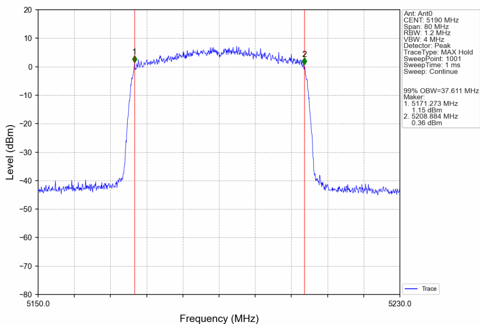
802.11ax(HEW40)_LCH_5190MHz_RU484_Left_Ant0_NTNV
