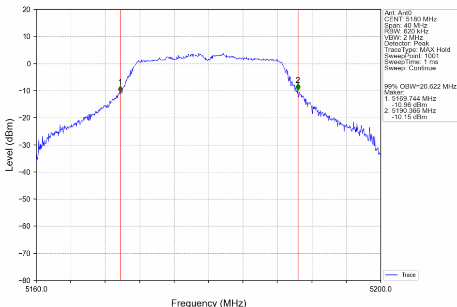
802.11ac(VHT20)_LCH_5180MHz_Ant0_NTNV
