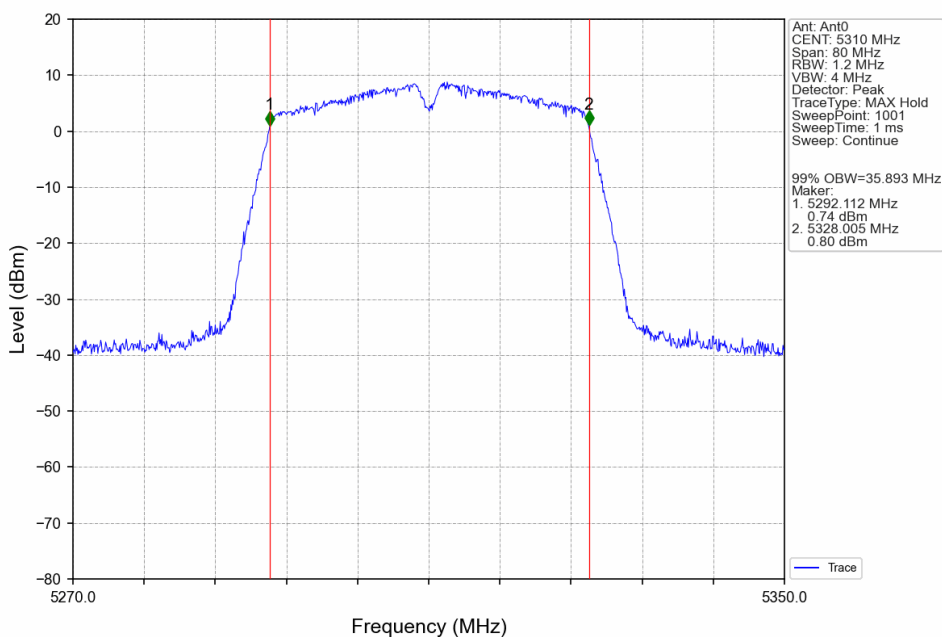
802.11n(HT40)_HCH_5310MHz_Ant0_NTNV
