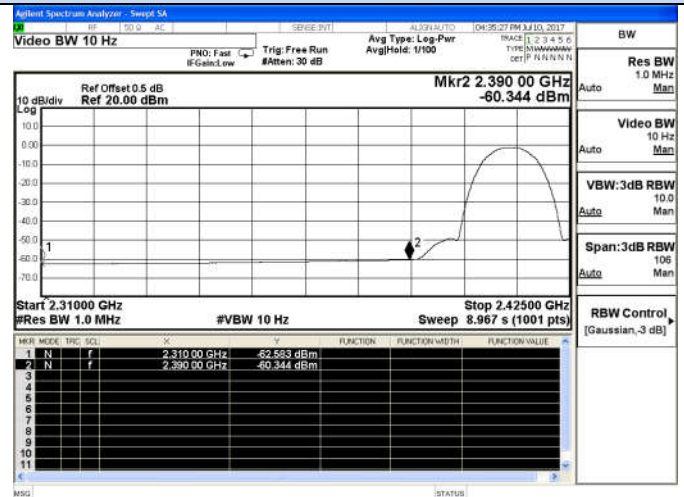
802.11b-Low channel(Average)
