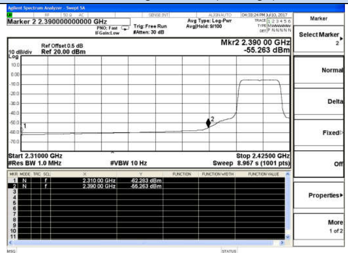
802.11g-Low channel(Average)
