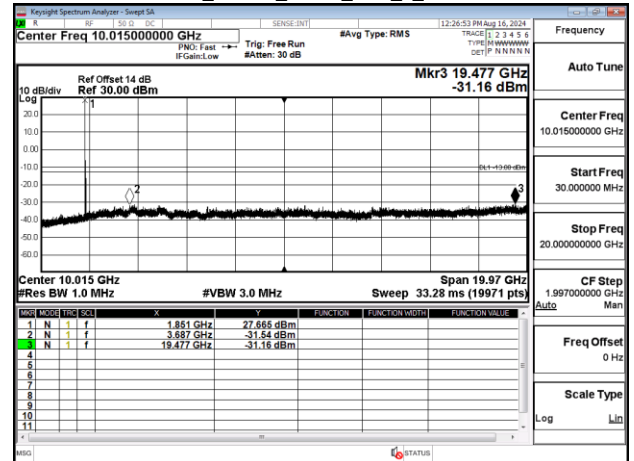
Band25_20MHz_QPSK_RB1_0_CH26140
