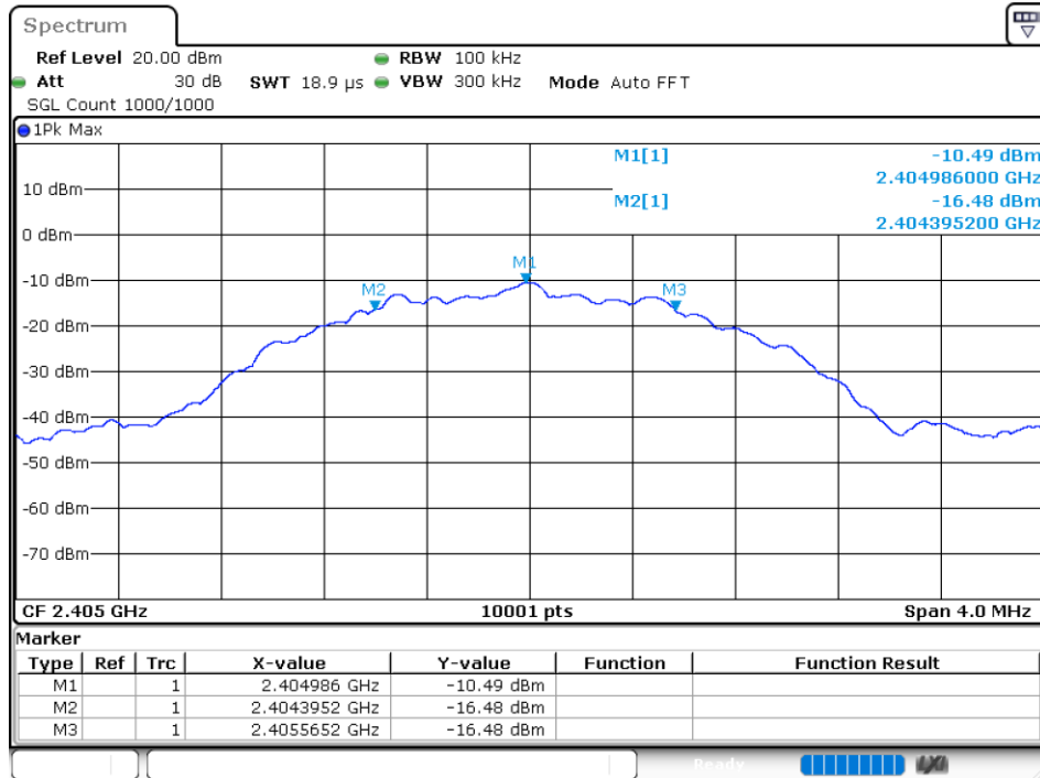
-6 dB BW NVNT GFSK 2405MHz Ant1
