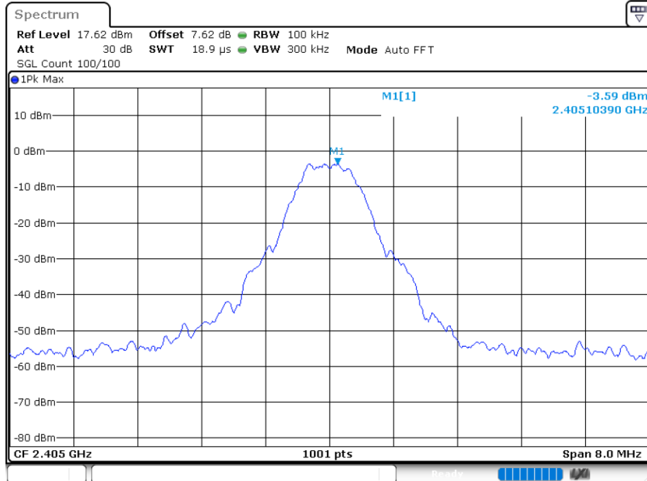
Band Edge NVNT GFSK 2405MHz Ant1 Ref
