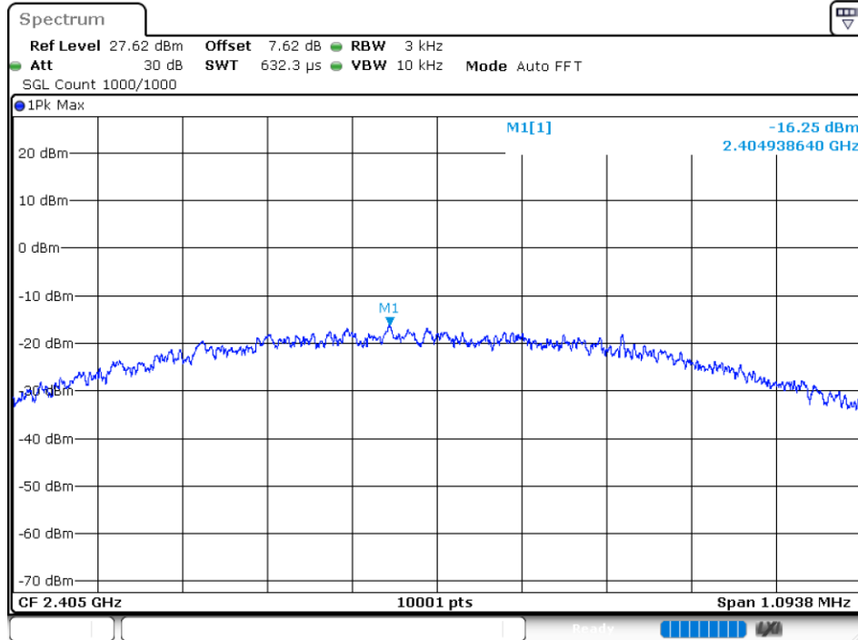
PSD NVNT GFSK 2405MHz Ant1
