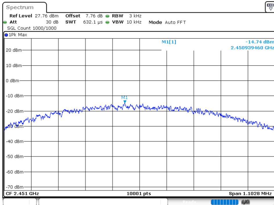
PSD NVNT GFSK 2451MHz Ant1
