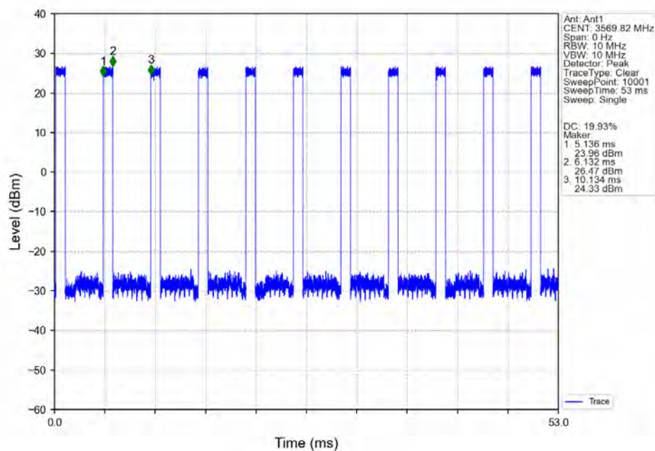
n48_30kHz_SISO_NTNV_40MHz_CP-OFDM QPSK_3570MHz_Inner_Full_Ant1
