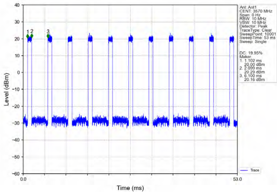
n48_30kHz_SISO_NTNV_40MHz_CP-OFDM QPSK_3570MHz_Inner_Full_Ant1
