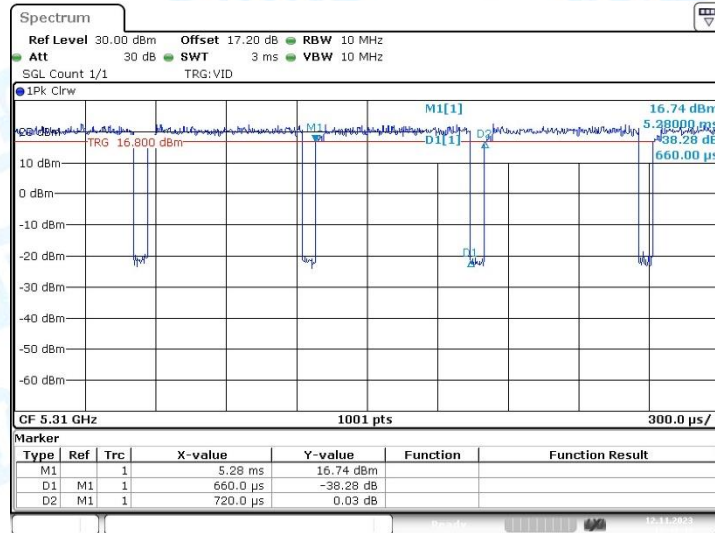
11AC40MIMO_Ant2_5310
