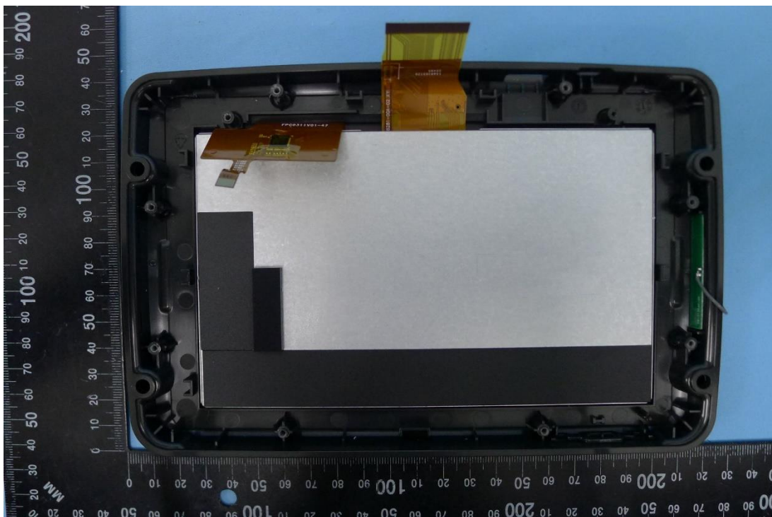
(10) EUT Photo
