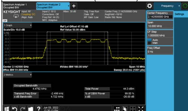
Ch 428500 (2142.5MHz)
