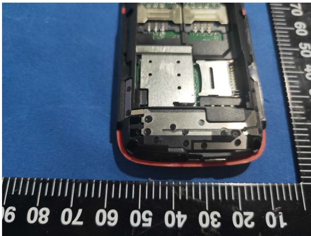
GSM Antenna
