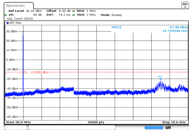
20MHz_Low_QPSK_1@0 -21.38dBm
