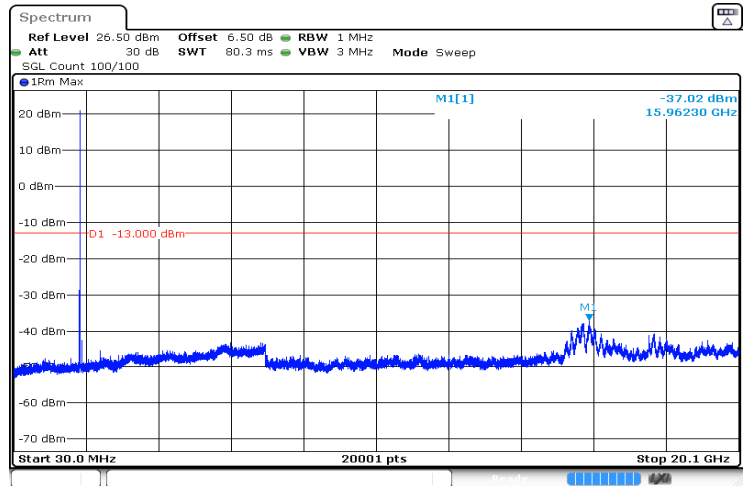
3MHz_Low_QPSK_15@0 -37.02 dBm
