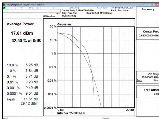
PTAR B41 20M CH41490 QPSK
