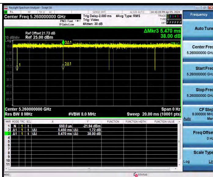
11AX20MIMO_Ant6_5260
