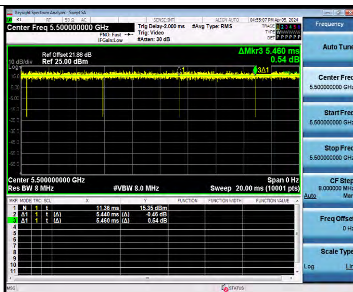
11AX20MIMO_Ant6_5500
