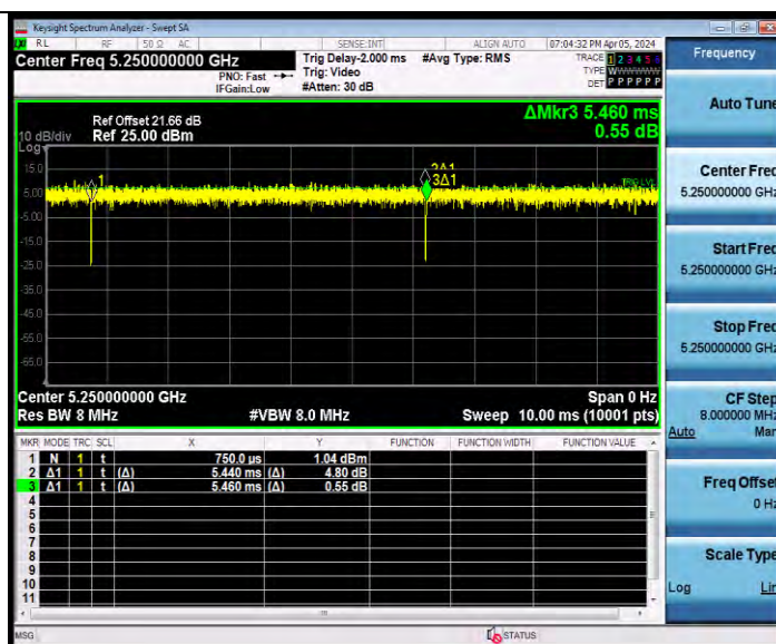
11AX160MIMO_Ant6_5250
