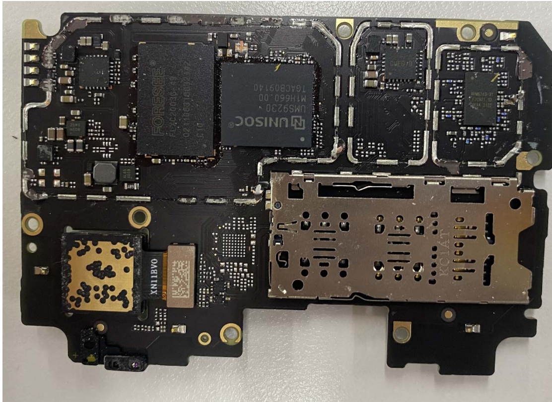
IC Details 1
