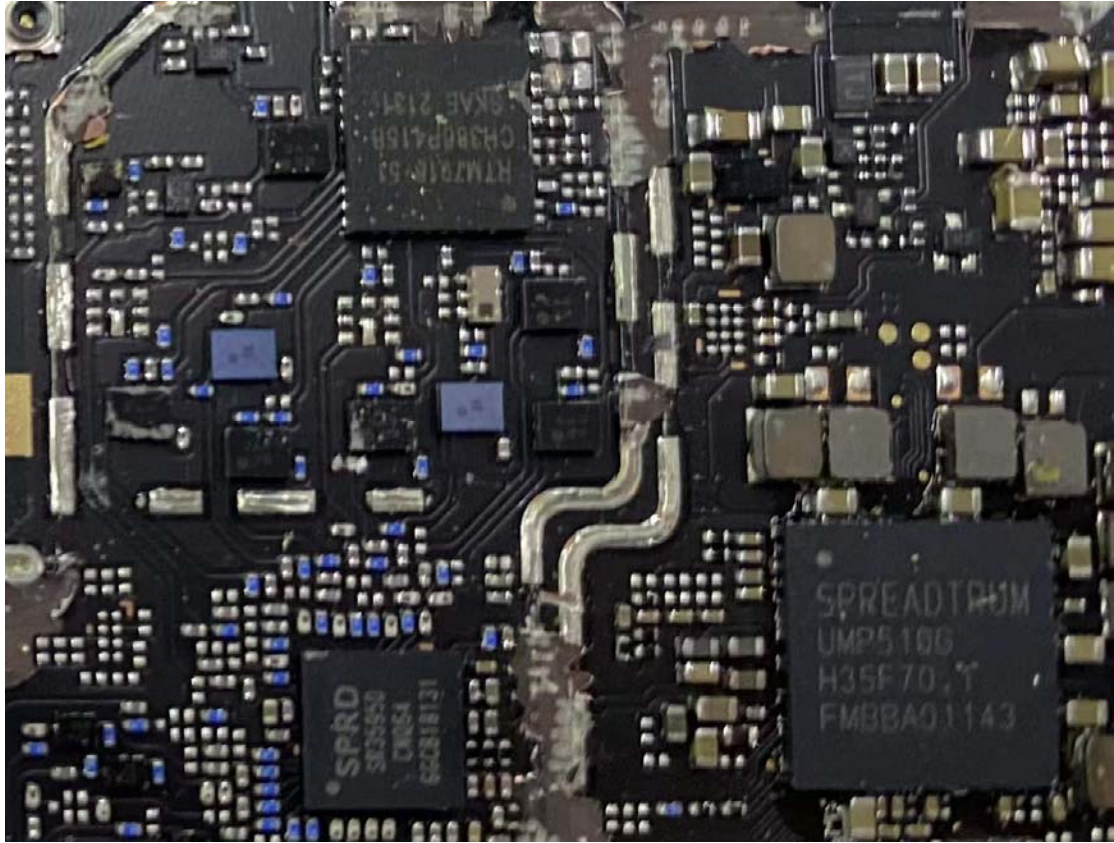
IC Details 9
