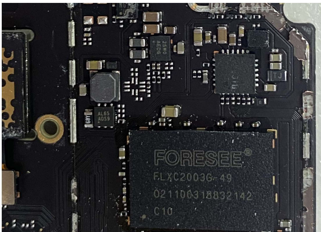
IC Details 6
