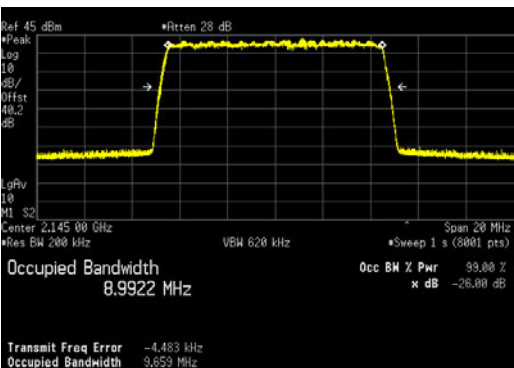
LTE10_16QAM
