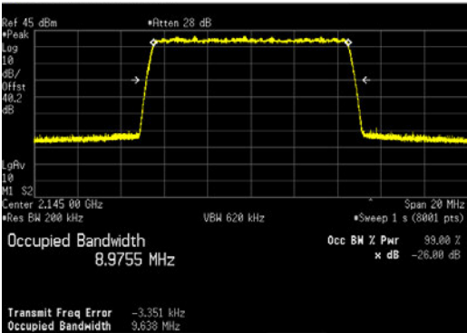
LTE10_QPSK
