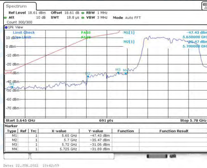
11N40MIMO_Ant2_Low_5755_Peak
