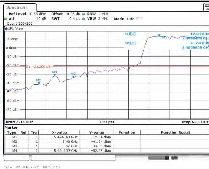
11N20MIMO_Ant1_Low_5500_Peak
