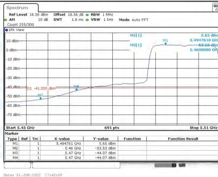
11A_Ant1_Low_5500_AV
