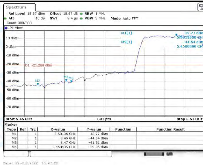
11AC20MIMO_Ant2_Low_5500_Peak
