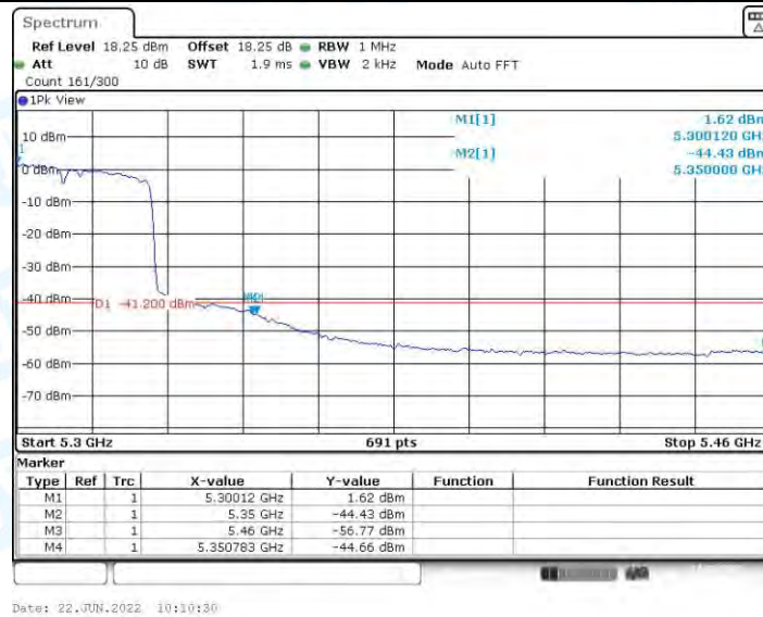
11N40MIMO_Ant2_High_5310_AV
