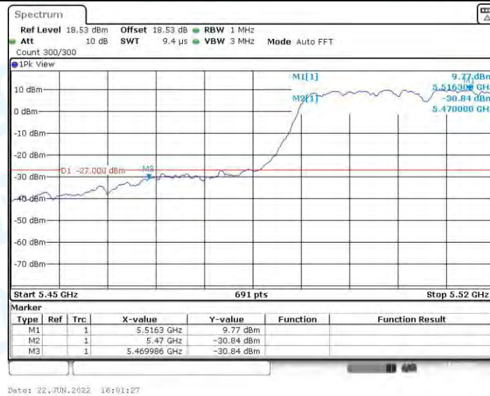
11AC40MIMO_Ant1_Low_5510
