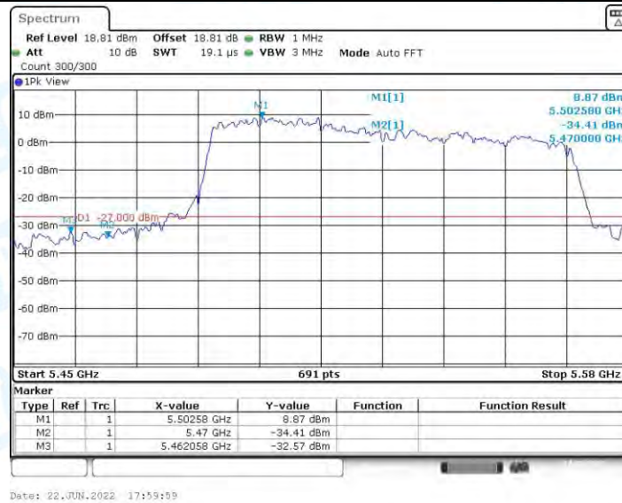
11AC80MIMO_Ant2_Low_5530
