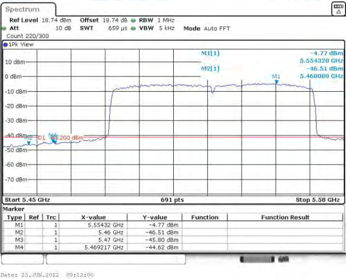
11AC80MIMO_Ant1_Low_5530_AV
