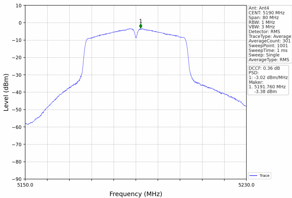
802.11n(HT40)_LCH_5190MHz_Ant4_NTNV
