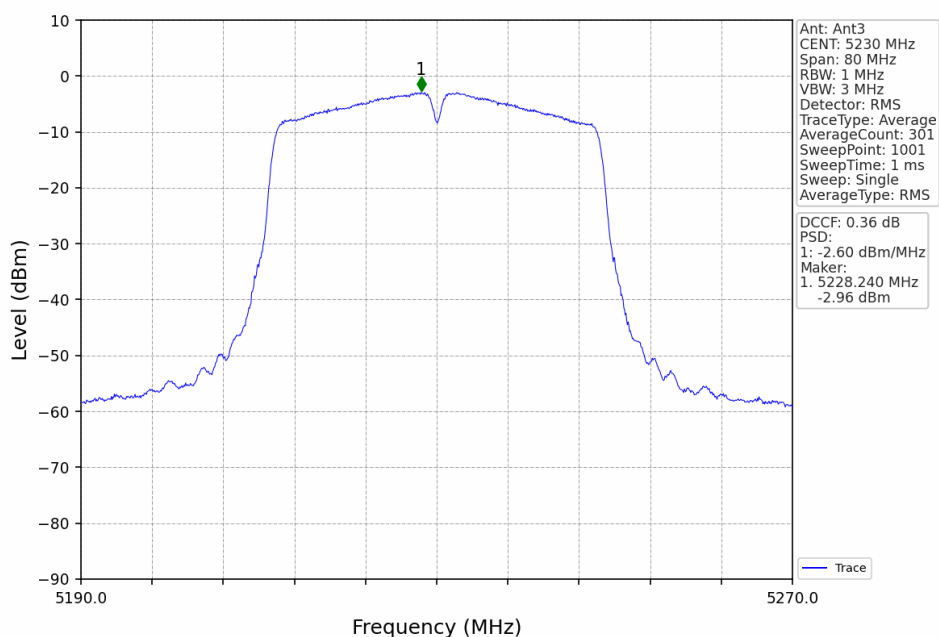
802.11n(HT40)_HCH_5230MHz_Ant3_NTNV
