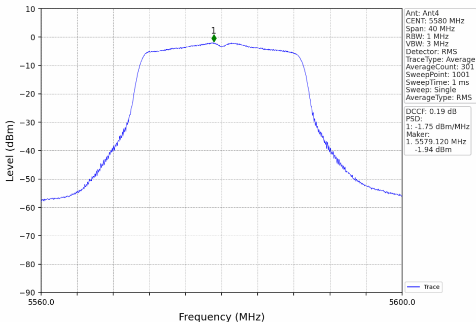
802.11n(HT20)_MCH_5580MHz_Ant4_NTNV
