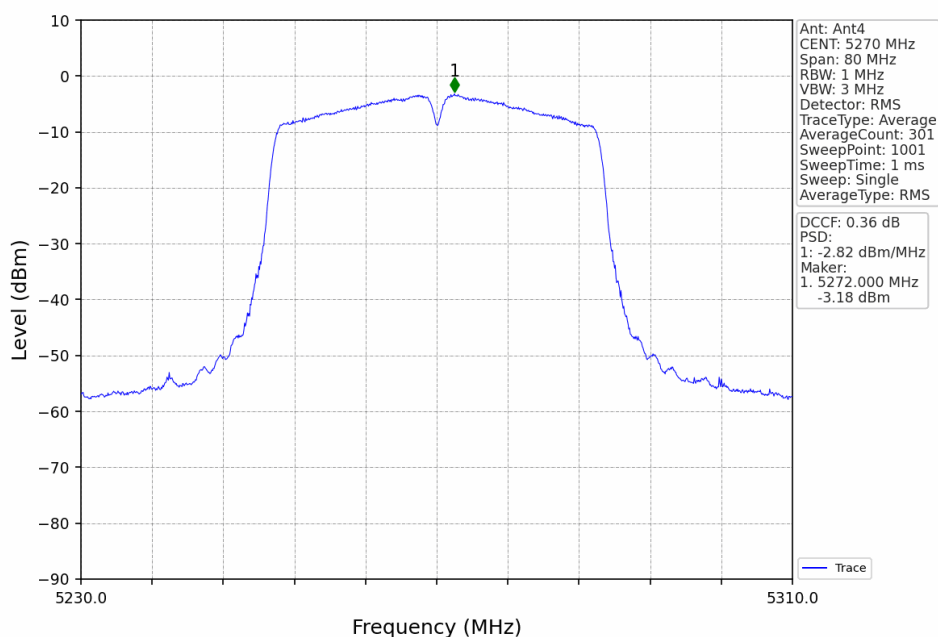
802.11n(HT40)_LCH_5270MHz_Ant4_NTNV
