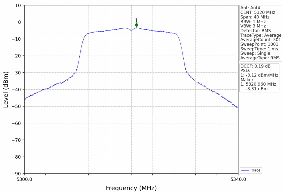
802.11n(HT20)_HCH_5320MHz_Ant4_NTNV
