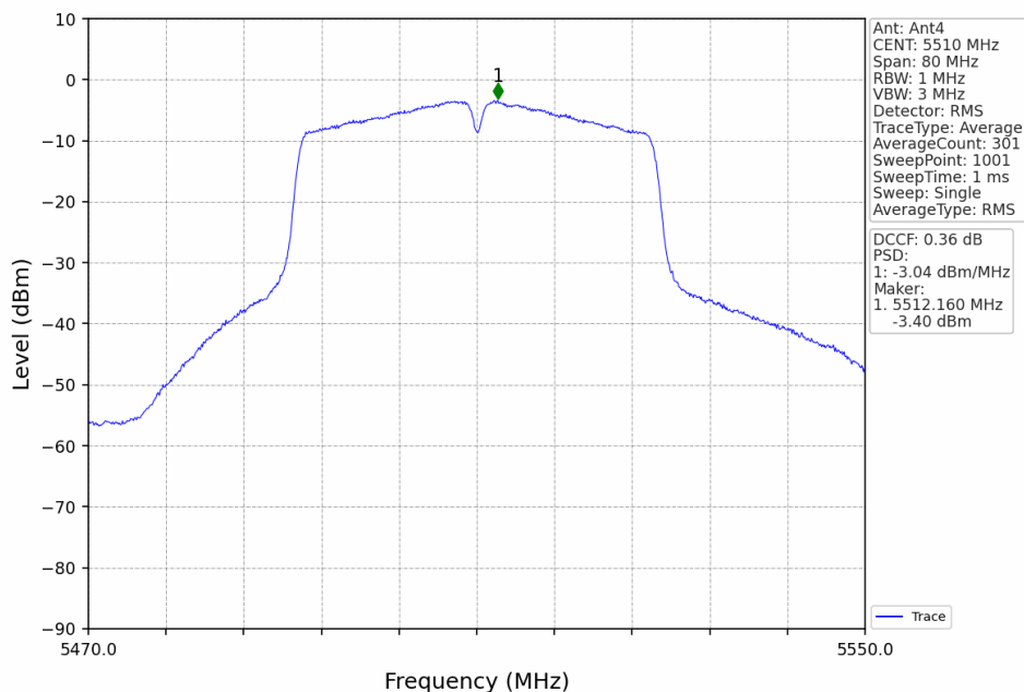
802.11n(HT40)_LCH_5510MHz_Ant4_NTNV
