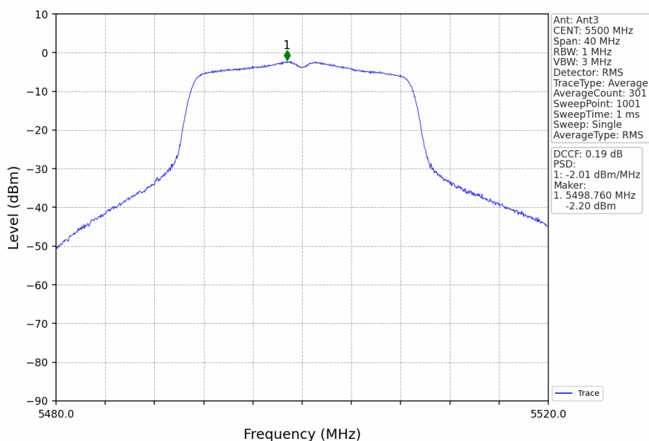
802.11n(HT20)_LCH_5500MHz_Ant3_NTNV
