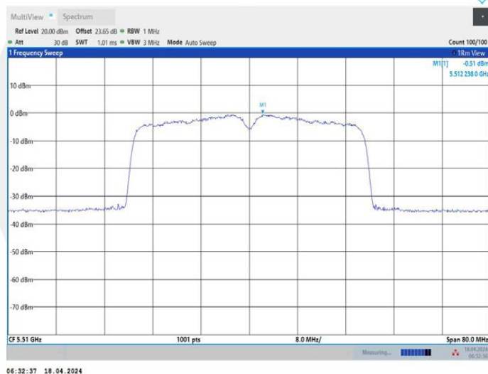
11AX40MIMO_Ant2_5510
