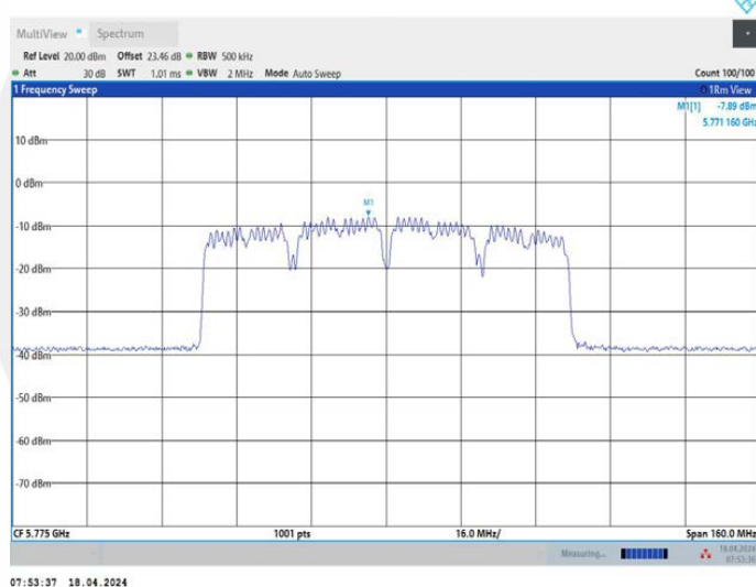
11AX80MIMO_Ant2_5775
