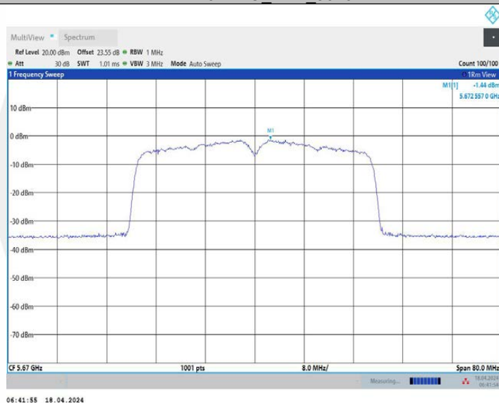
11AX40MIMO_Ant2_5670
