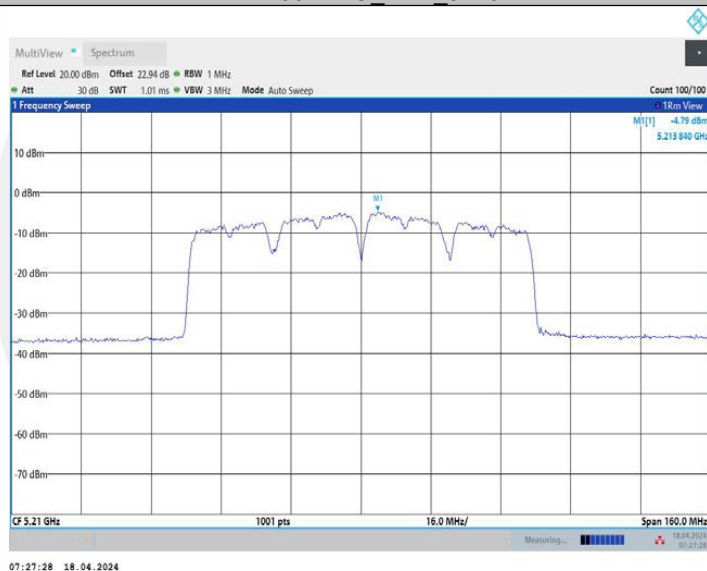
11AX80MIMO_Ant2_5210
