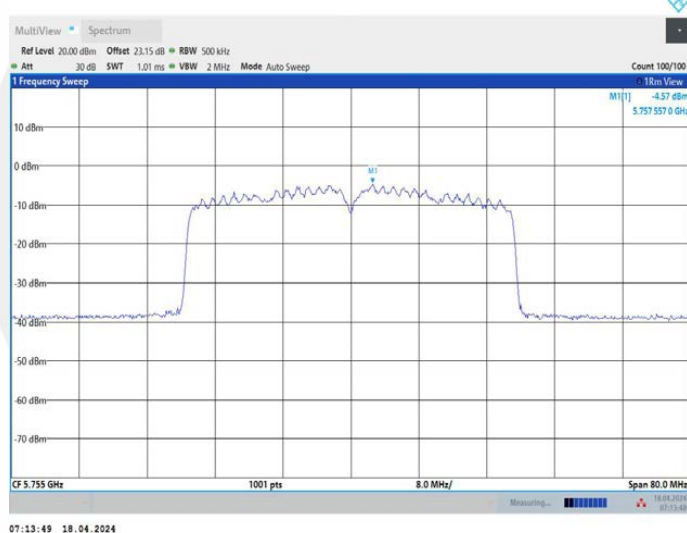
11AX40MIMO_Ant2_5755
