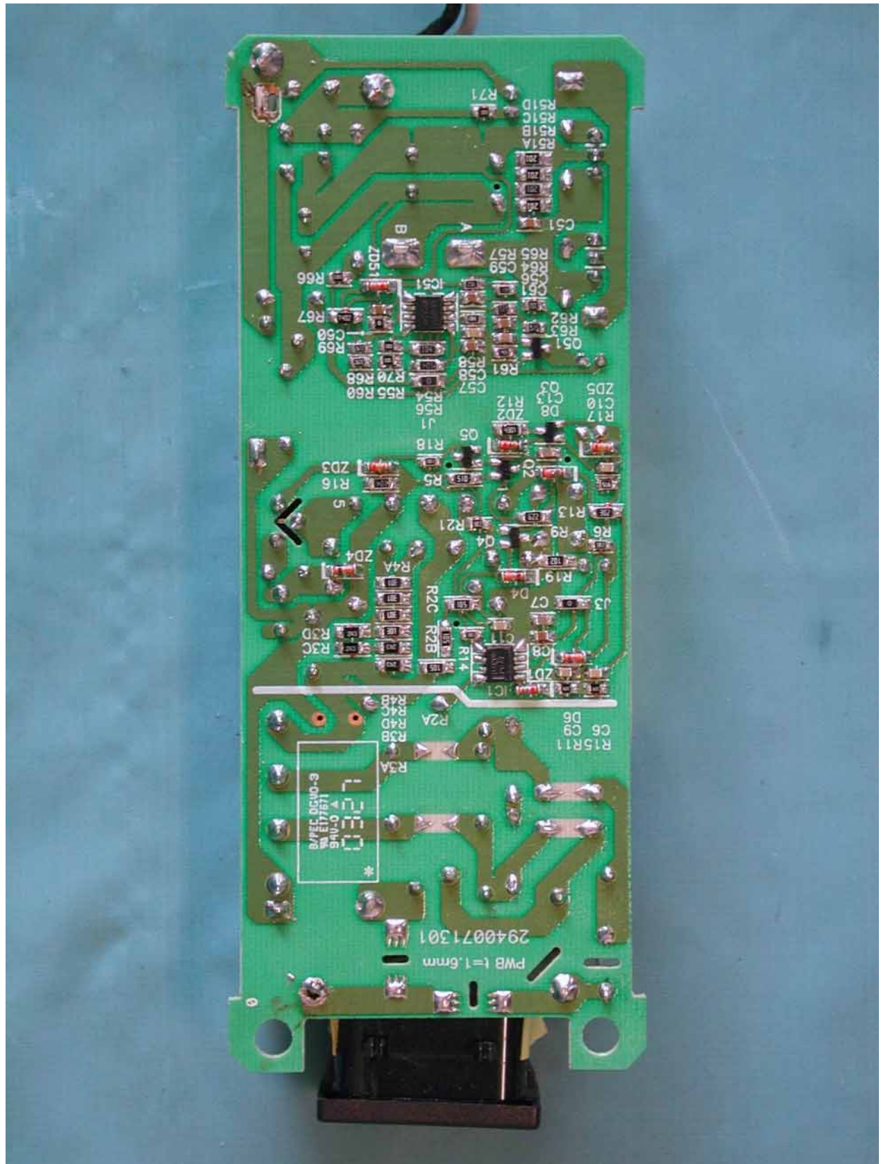
PCB Layout (Delta)
