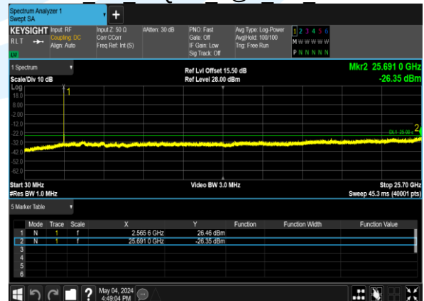
B7_5M 16QAM 1@0 CH 21425
