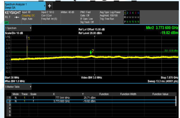
B13 5M 16QAM 1@0 CH 23205
