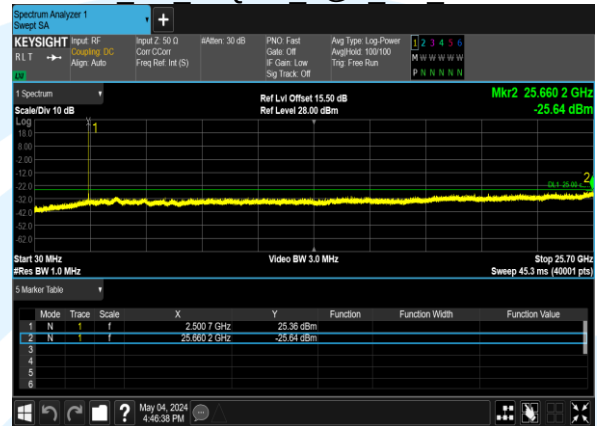
B7_5M 16QAM 1@0 CH 21100
