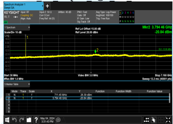
B66 20M 16QAM 1@0 CH 132072
