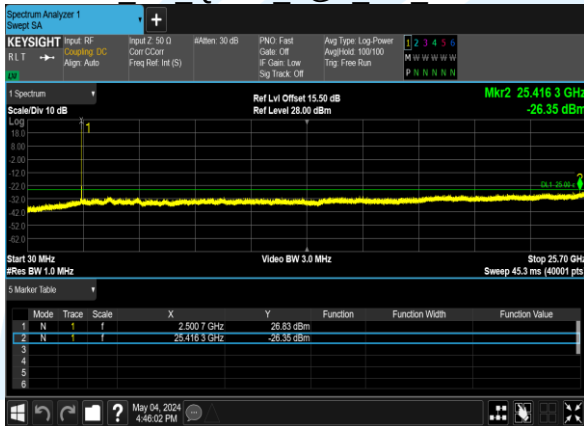
B7_5M QPSK 1@0 CH 21100
