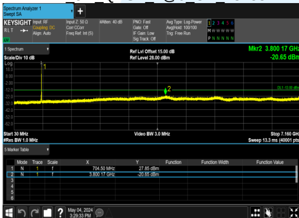
B17 5M QPSK 1@0 CH 23755
