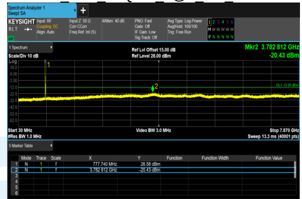
B13 10M 16QAM 1@0 CH 23230
