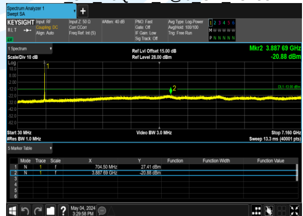
B17 5M 16QAM 1@0 CH 23755
