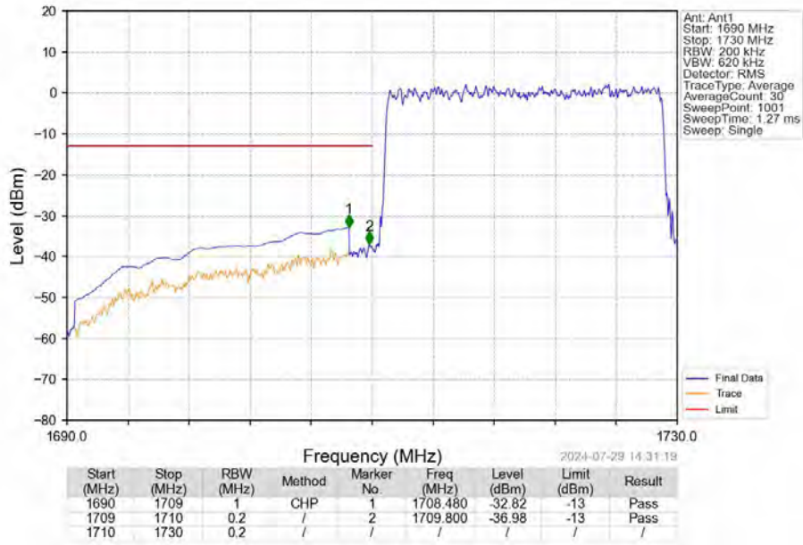
Band66_20MHz_16QAM_LCH_1720MHz_RB_100_0_NTNV
