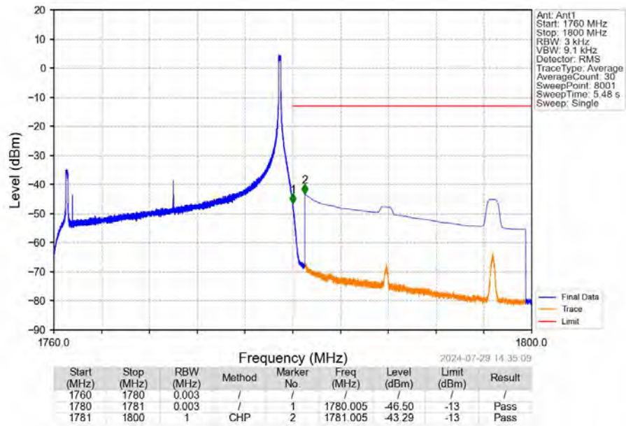
Band66_20MHz_QPSK_HCH_1770MHz_RB_1_99_NTNV
