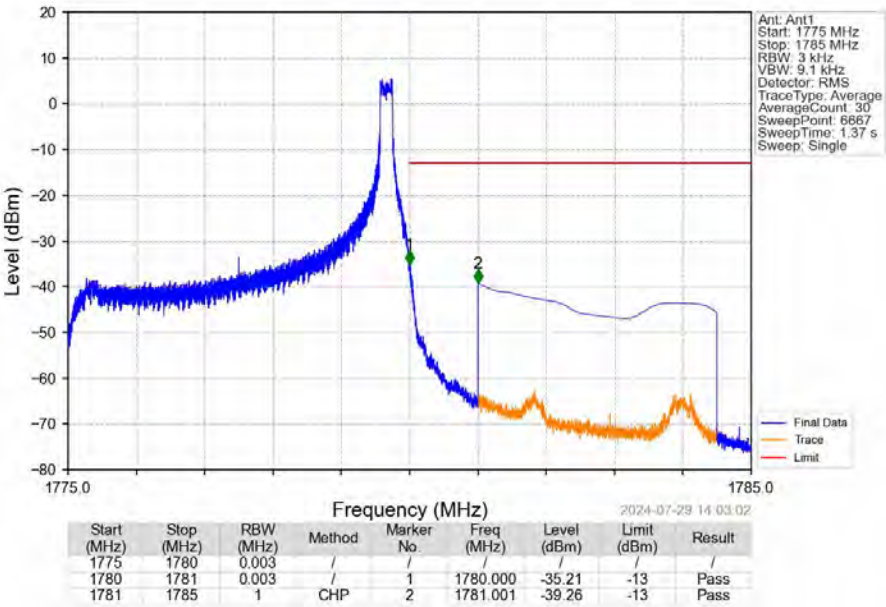
Band66_5MHz_QPSK_HCH_1777.5MHz_RB_1_24_NTNV
