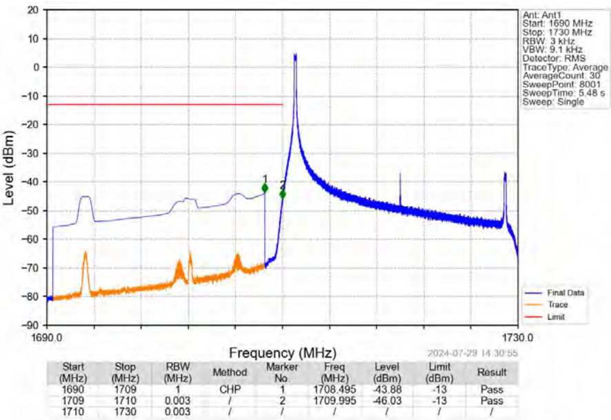
Band66_20MHz_16QAM_LCH_1720MHz_RB_1_0_NTNV
