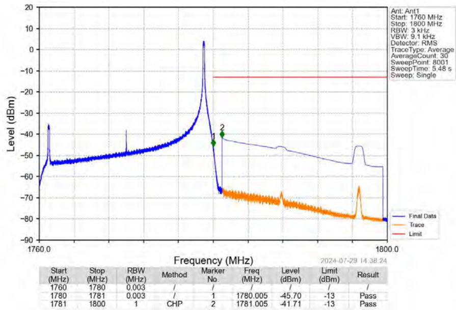
Band66_20MHz_16QAM_HCH_1770MHz_RB_1_99_NTNV
