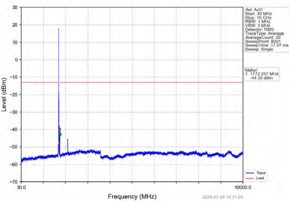
Band66_20MHz_16QAM_LCH_1720MHz_RB_1_0_NTNV
