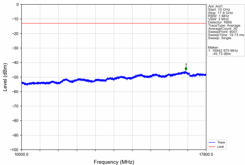
Band66_20MHz_16QAM_LCH_1720MHz_RB_100_0 NTN
