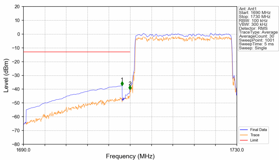
Band66_20MHz_16QAM_LCH_1720MHz_RB_100_0 NTN
