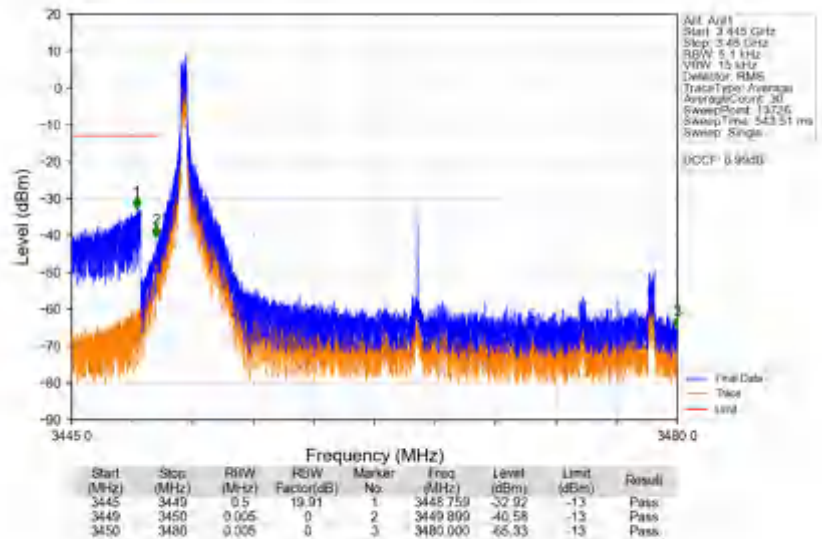
n78e_30kHz_SISO_NTNV_30MHz_DFT-s-OFDM_QPSK_3465MHz_Inner_1RB_Left
