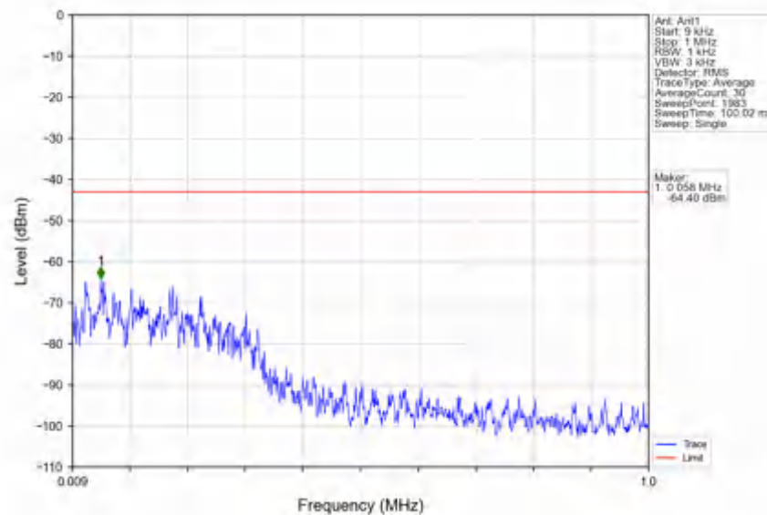
n78e_30kHz_SISO_NTV_30MHz_CP-OFDM QPSK_3465MHz_Inner_1RB_Left
