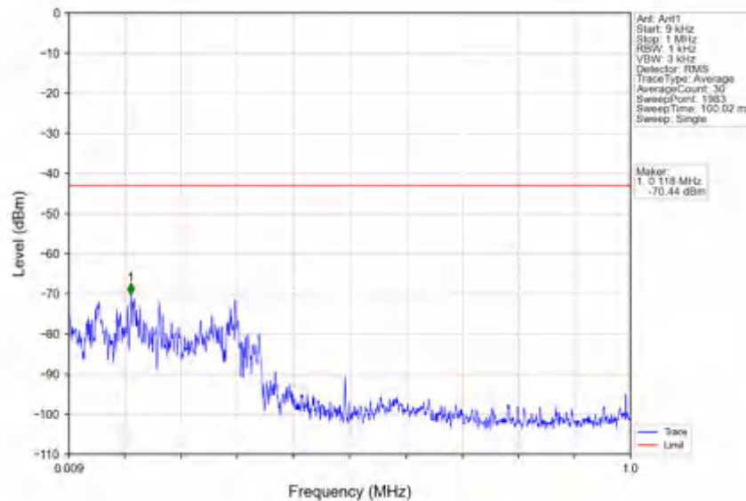
n78e_30kHz_SISO_NTNV_30MHz_DFT-s-OFDM_PI/2_BPSK_3465MHz_Inner_1RB_Left
