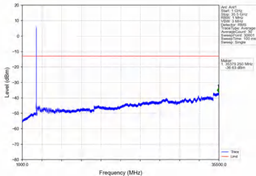
n78e_30kHz_SISO_NTNV_30MHz_DFT-s-OFDM_QPSK_3465MHz_Inner_1RB_Left
