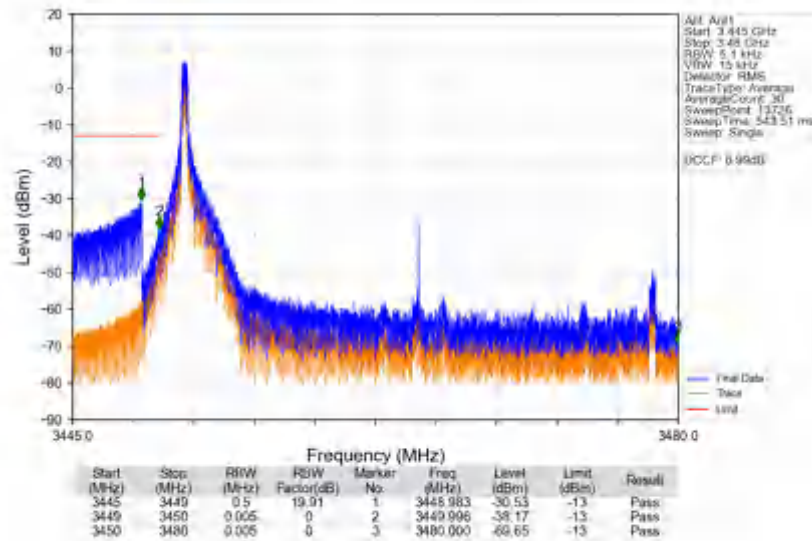
n78e_30kHz_SISO_NTNV_30MHz_DFT-s-OFDM_PI/2_BPSK_3465MHz_Inner_1RB_Left
