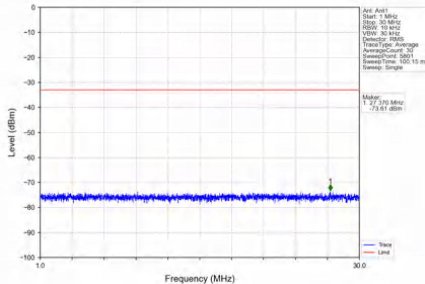
n78e_30kHz_SISO_NTV_30MHz_DFT-s-OFDM QPSK_3465MHz_Inner_1RB_Left
