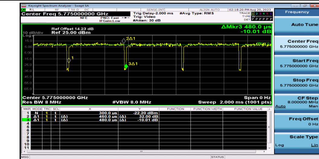
NTNV-11AC80SISO-Ant1-5775
