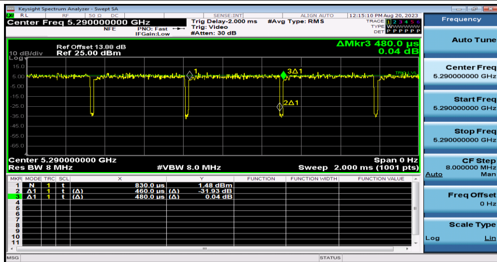
NTNV-11AC80SISO-Ant1-5290
