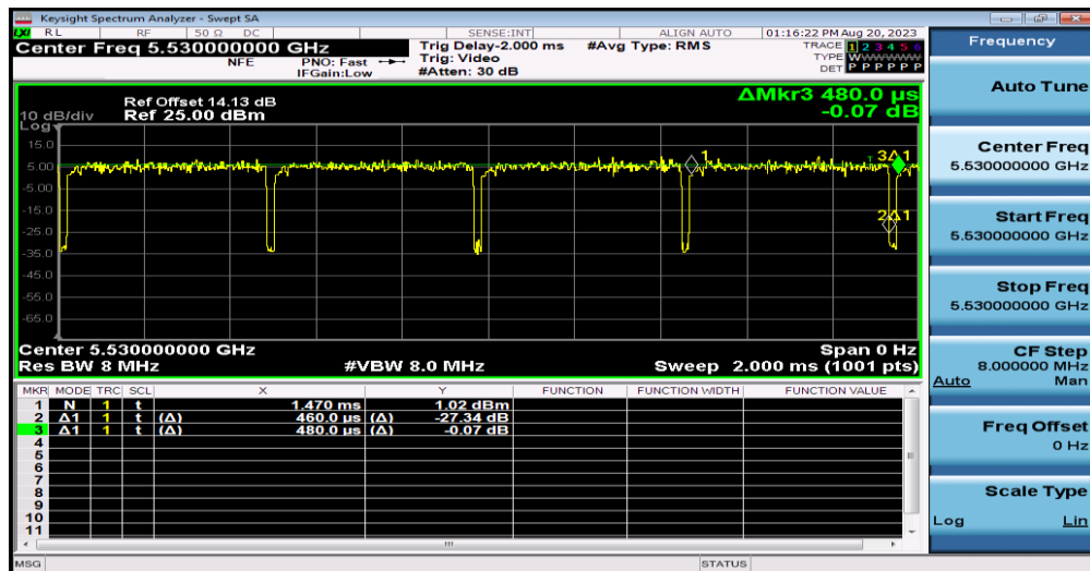
NTNV-11AC80SISO-Ant1-5530
