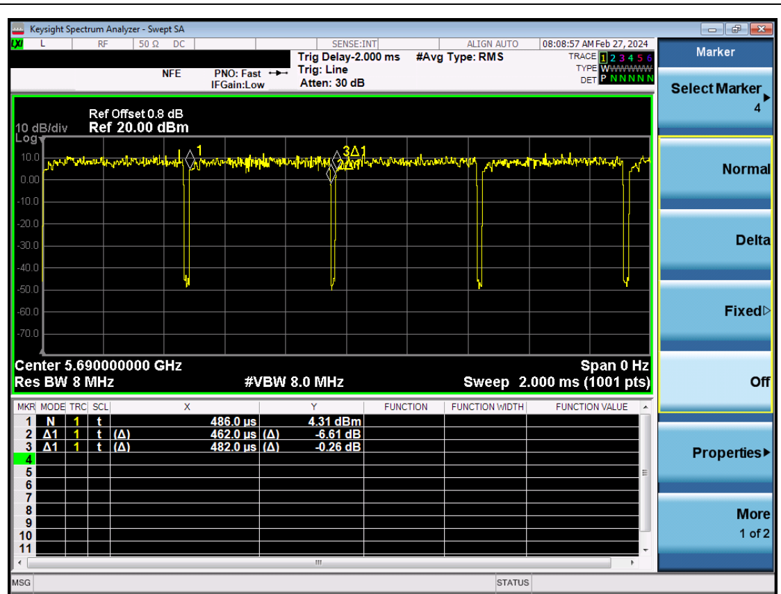
NTNV-11AC80SISO-Ant1-5690
