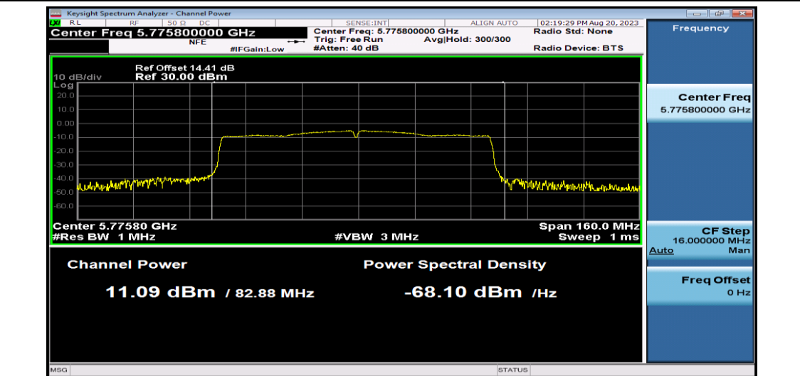
11AC80SISO-Ant1-5775
