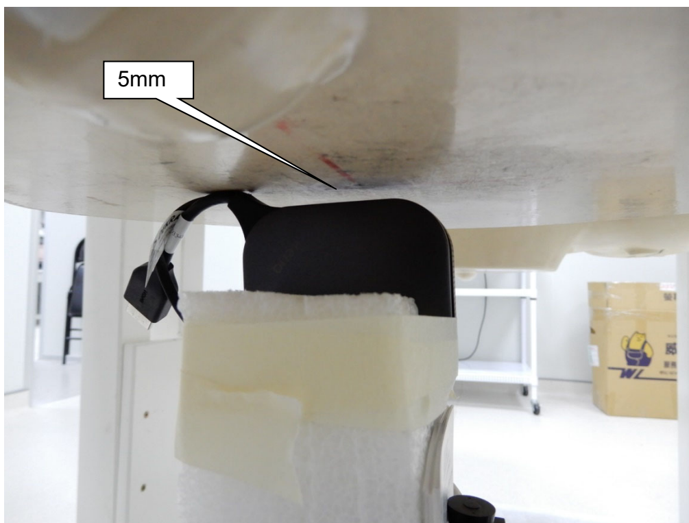
EUT Left-side_5mm
