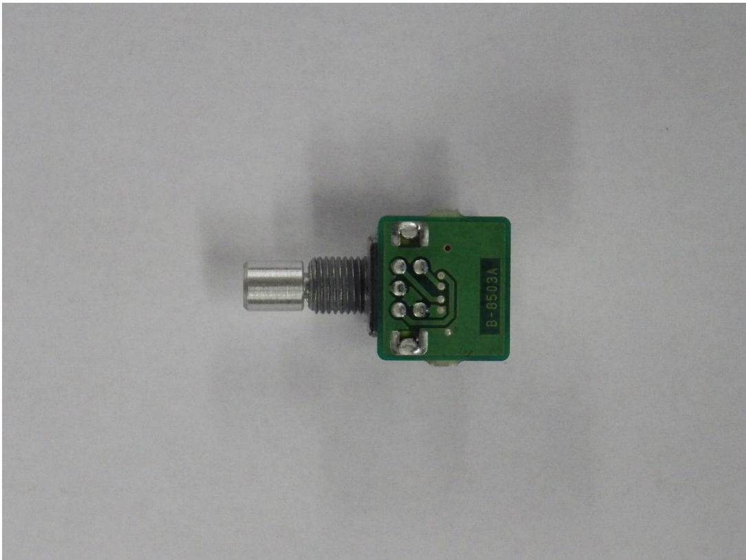
ENC-3_SIDE_B
