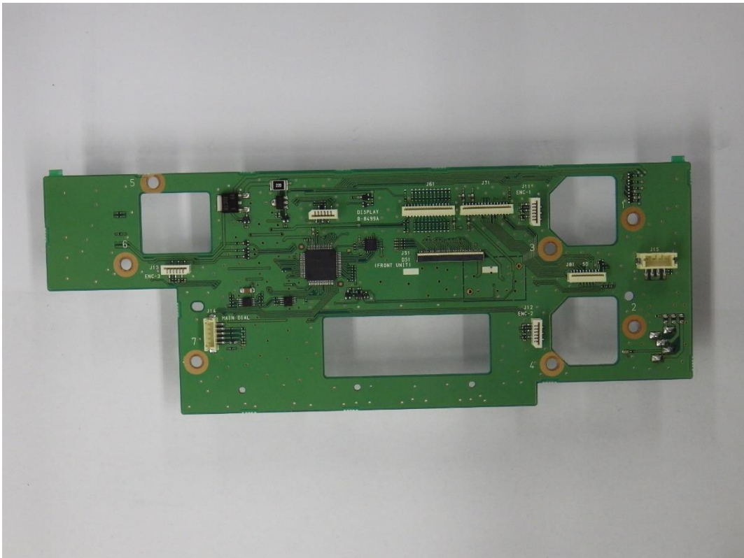
DISPLAY_SIDE_B
