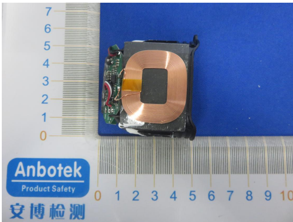
RX ANT
