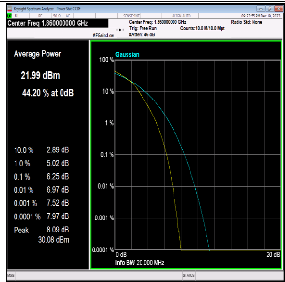
Band2-20MHz-16QAM-18700-100RB#0-PASS
