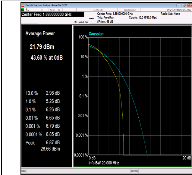
Band2-20MHz-64QAM-18900-1RB#0-PASS
