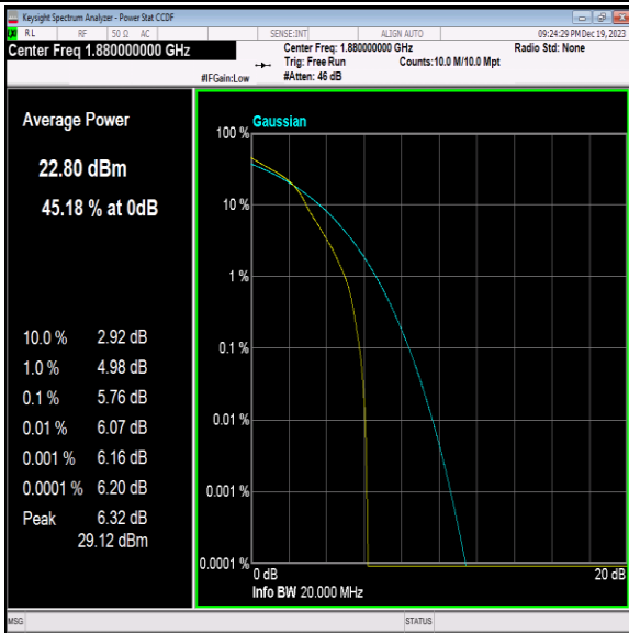
Band2-20MHz-16QAM-18900-1RB#0-PASS
