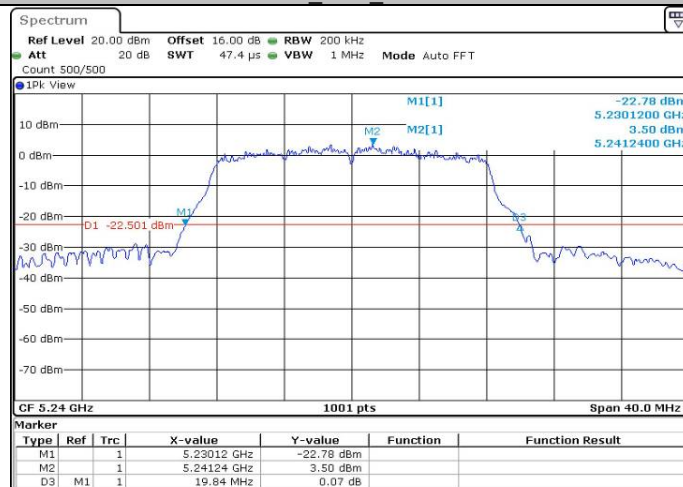
11A_Ant1_5240
