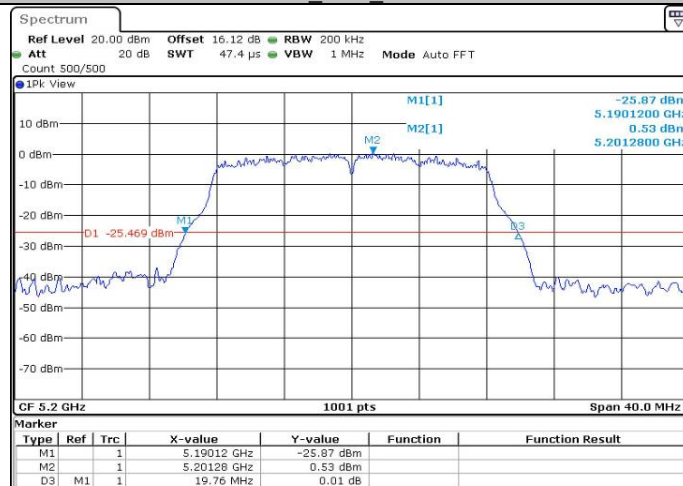
11A_Ant1_5200
