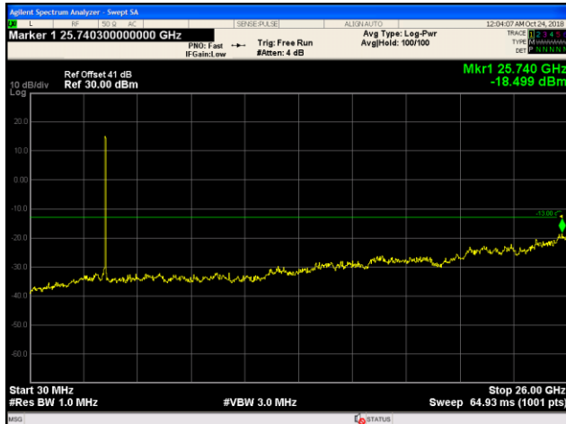
30MHz~26GHz
