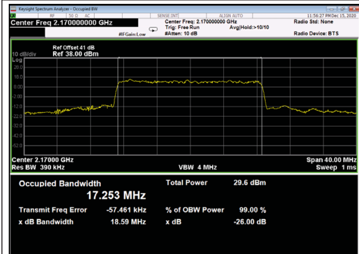
Figure 635: 64QAM 20MHz B.W.; 2170.0MHz, 60kHz - Output
