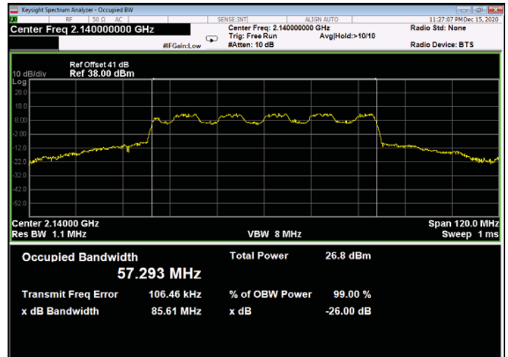
Figure 598: 16QAM 60MHz B.W.; 2140.0MHz, 60kHz - Output
