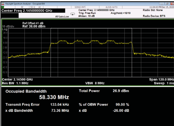
Figure 599: 16QAM 60MHz B.W.; 2145.0MHz, 30kHz - Output
