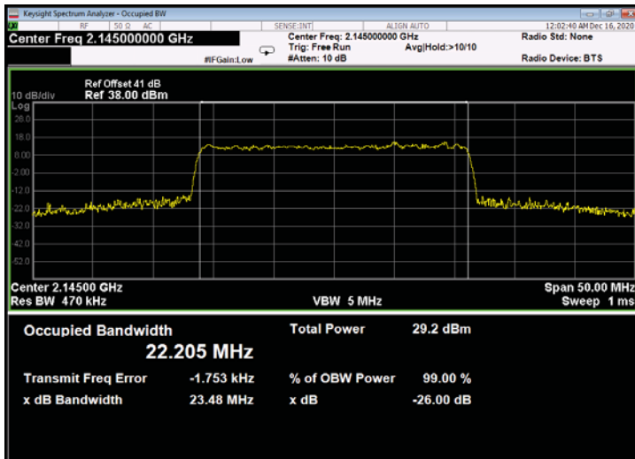
Figure 641: 64QAM 25MHz B.W.; 2145.0MHz, 60kHz - Output
