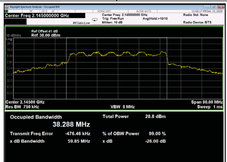
Figure 584: 16QAM 40MHz B.W.; 2145.0MHz, 60kHz - Output
