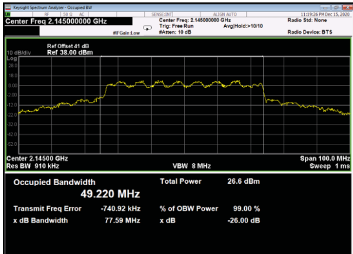
Figure 593: 16QAM 50MHz B.W.; 2145.0MHz, 60kHz - Output
