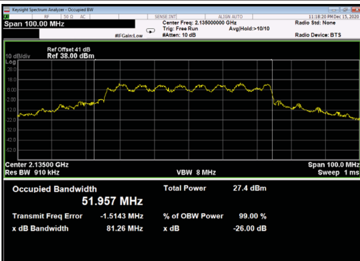
Figure 589: 16QAM 50MHz B.W.; 2135.0MHz, 30kHz - Output
