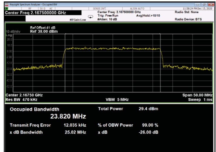
Figure 642: 64QAM 25MHz B.W.; 2167.5MHz, 15kHz - Output
