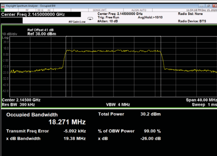
Figure 631: 64QAM 20MHz B.W.; 2145.0MHz, 30kHz - Output
