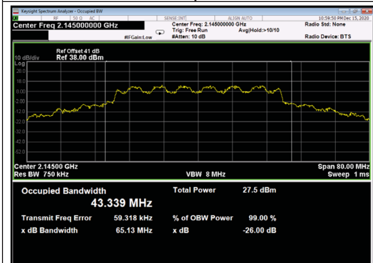
Figure 583: 16QAM 40MHz B.W.; 2145.0MHz, 30kHz - Output
