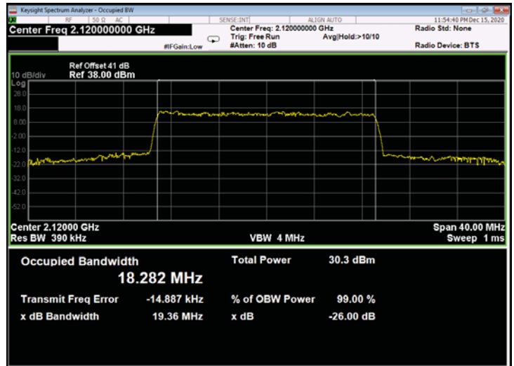
Figure 628: 64QAM 20MHz B.W.; 2120.0MHz, 30kHz - Output
