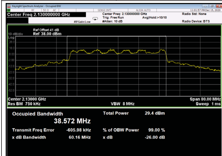
Figure 581: 16QAM 40MHz B.W.; 2130.0MHz, 60kHz - Output
