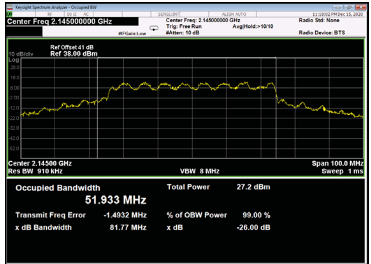
Figure 592: 16QAM 50MHz B.W.; 2145.0MHz, 30kHz - Output
