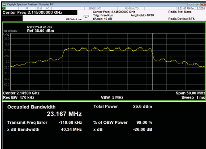
Figure 575: 16QAM 25MHz B.W.; 2145.0MHz, 60kHz - Output
