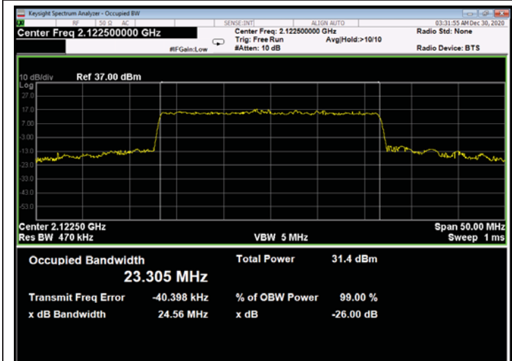
Figure 637: 64QAM 25MHz B.W.; 2122.5MHz, 30kHz - Output
