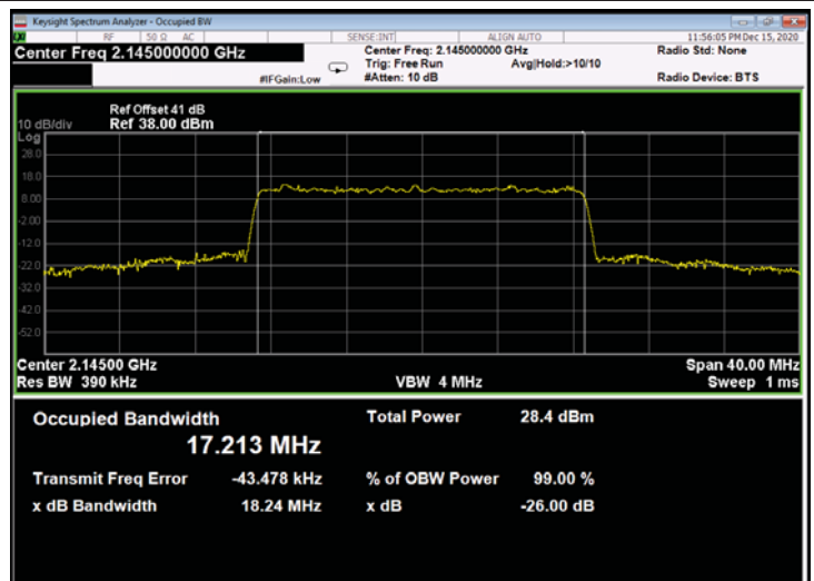
Figure 632: 64QAM 20MHz B.W.; 2145.0MHz, 60kHz - Output
