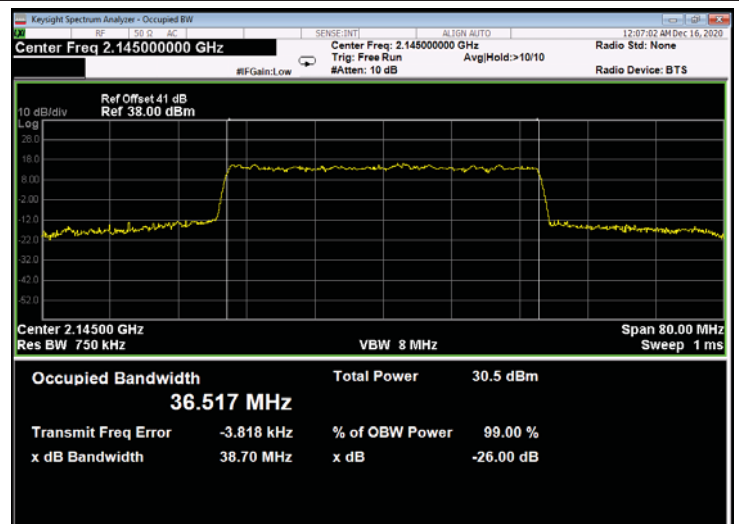
Figure 650: 64QAM 40MHz B.W.; 2145.0MHz, 60kHz - Output
