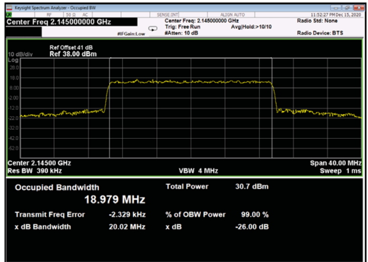
Figure 630: 64QAM 20MHz B.W.; 2145.0MHz, 15kHz - Output
