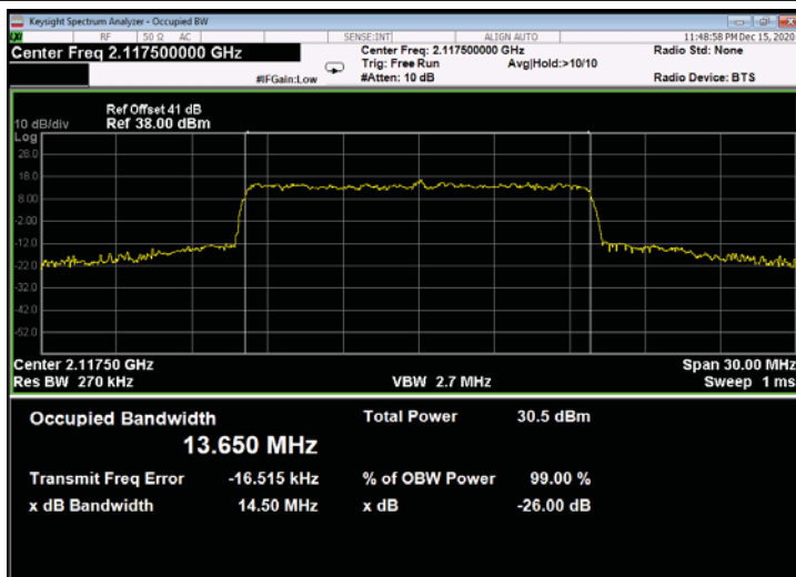
Figure 619: 64QAM 15MHz B.W.; 2117.5MHz, 30kHz - Output
