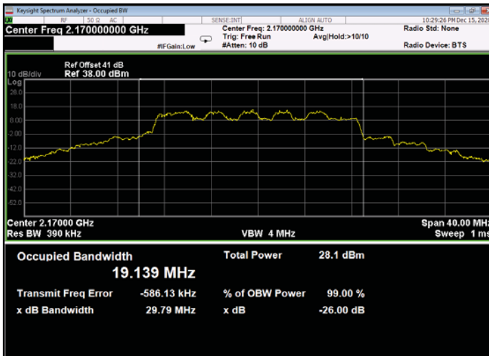
Figure 569: 16QAM 20MHz B.W.; 2170.0MHz, 60kHz - Output
