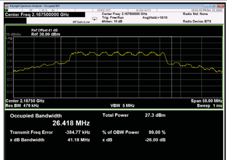
Figure 578: 16QAM 25MHz B.W.; 2167.5MHz, 60kHz - Output
