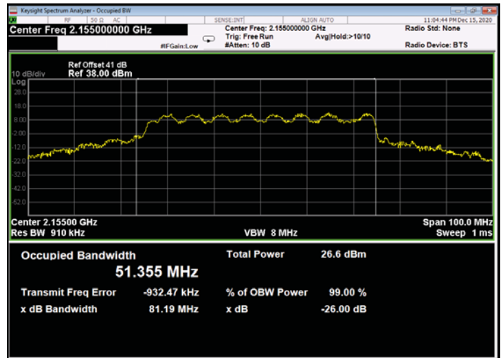
Figure 594: 16QAM 50MHz B.W.; 2155.0MHz, 15kHz - Output
