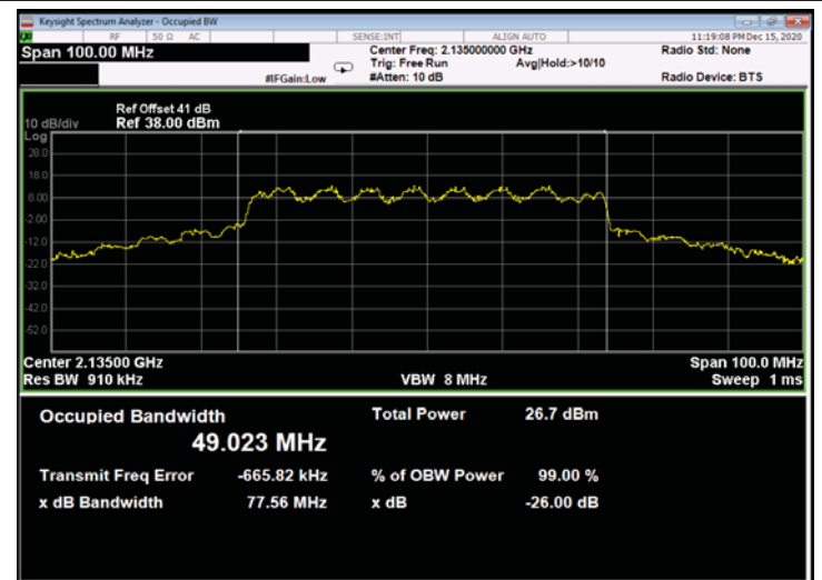
Figure 590: 16QAM 50MHz B.W.; 2135.0MHz, 60kHz - Output
