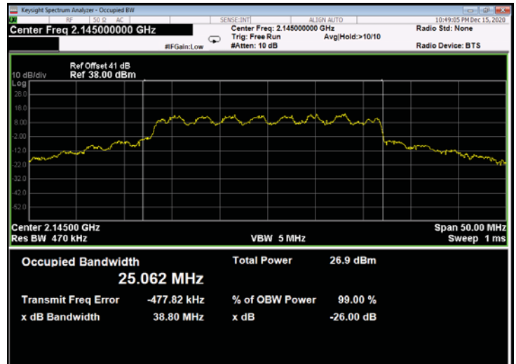
Figure 574: 16QAM 25MHz B.W.; 2145.0MHz, 30kHz - Output
