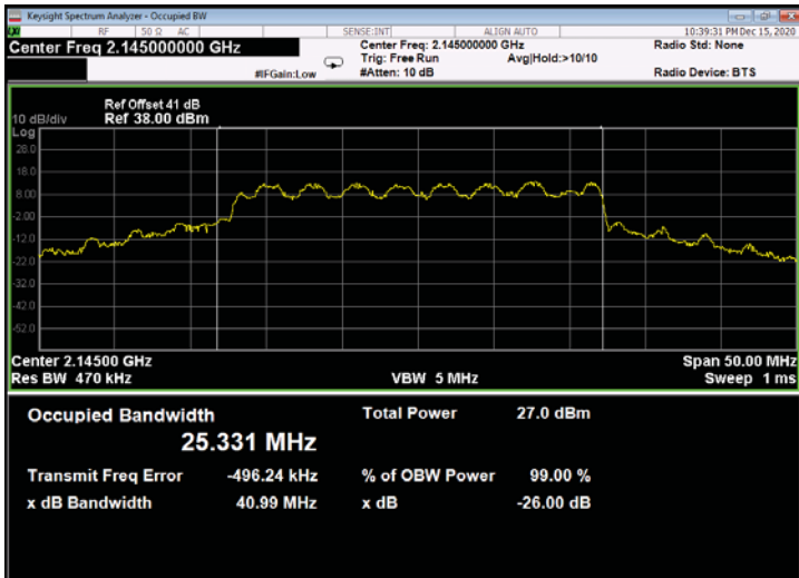
Figure 573: 16QAM 25MHz B.W.; 2145.0MHz, 15kHz - Output
