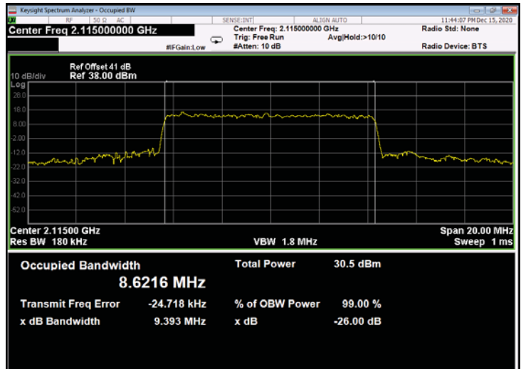
Figure 610: 64QAM 10MHz B.W.; 2115.00MHz, 30kHz - Output
