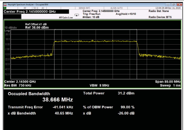
Figure 648: 64QAM 40MHz B.W.; 2145.0MHz, 15kHz - Output
