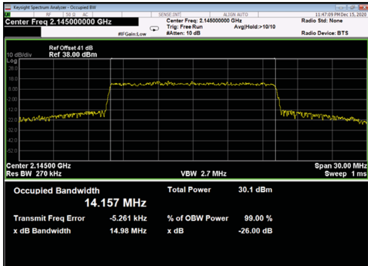
Figure 621: 64QAM 15MHz B.W.; 2145.0MHz, 15kHz - Output
