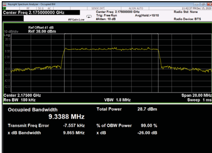
Figure 615: 64QAM 10MHz B.W.; 2175.0MHz, 15kHz - Output
