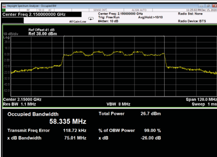
Figure 601: 16QAM 60MHz B.W.; 2150.0MHz, 30kHz - Output
