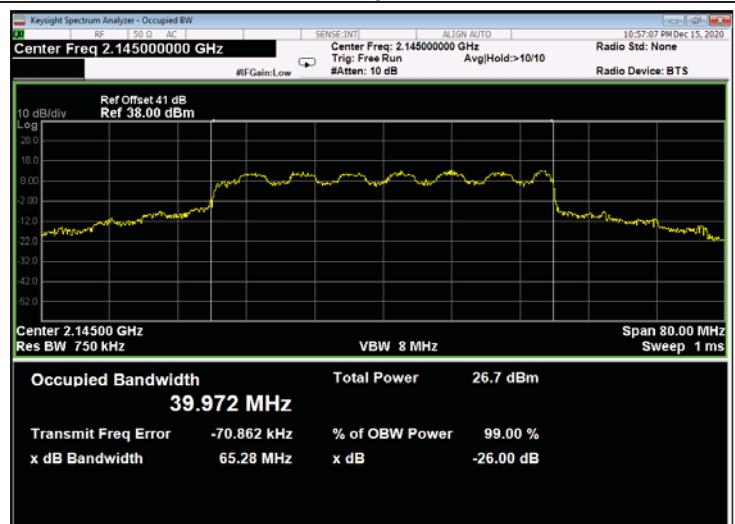
Figure 582: 16QAM 40MHz B.W.; 2145.0MHz, 15kHz - Output
