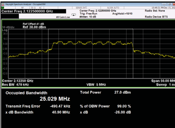
Figure 571: 16QAM 25MHz B.W.; 2122.5MHz, 30kHz - Output
