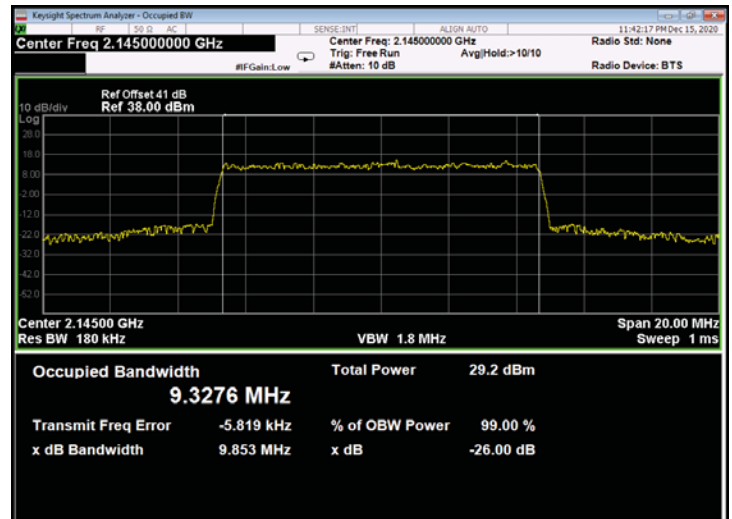
Figure 612: 64QAM 10MHz B.W.; 2145.00MHz, 15kHz - Output
