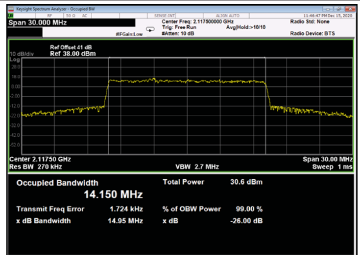
Figure 618: 64QAM 15MHz B.W.; 2117.5MHz, 15kHz - Output
