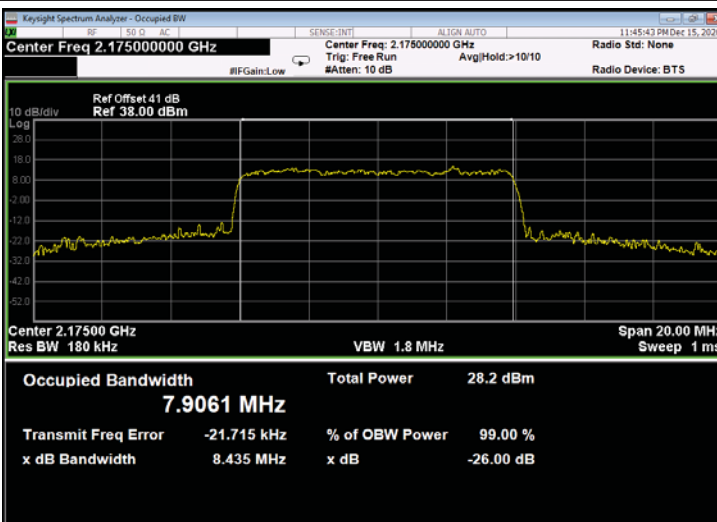
Figure 617: 64QAM 10MHz B.W.; 2175.0MHz, 60kHz - Output
