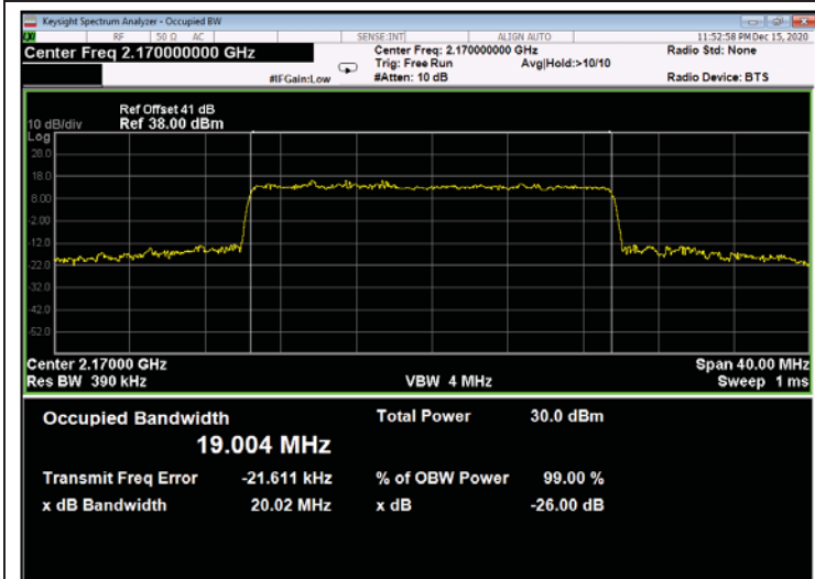
Figure 633: 64QAM 20MHz B.W.; 2170.0MHz, 15kHz - Output
