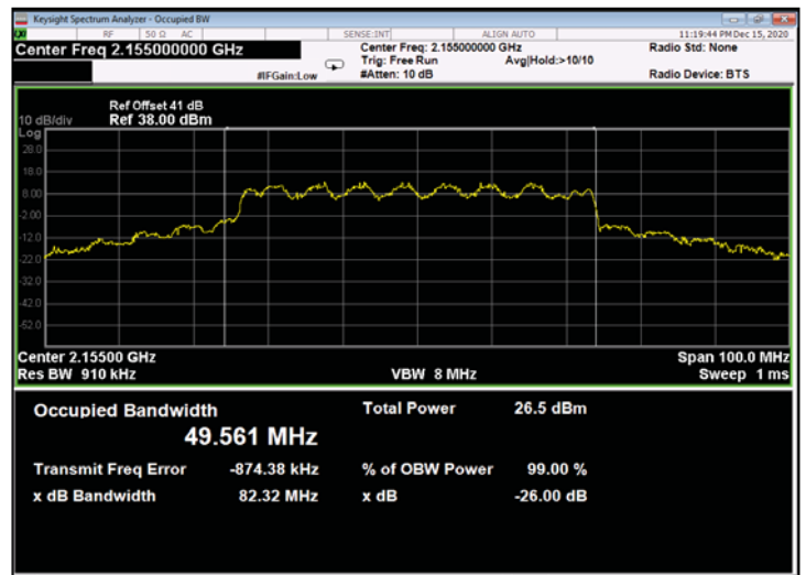
Figure 596: 16QAM 50MHz B.W.; 2155.0MHz, 60kHz - Output
