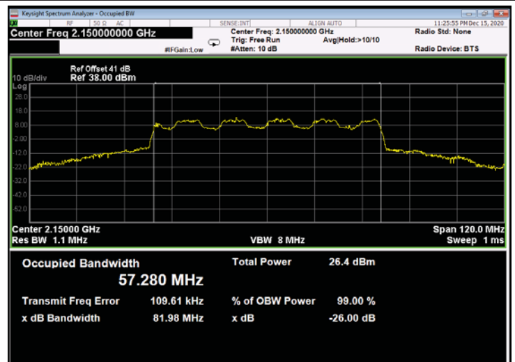
Figure 602: 16QAM 60MHz B.W.; 2150.0MHz, 60kHz - Output
