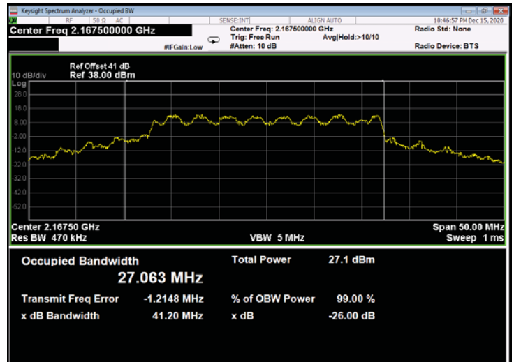
Figure 576: 16QAM 25MHz B.W.; 2167.5MHz, 15kHz - Output
