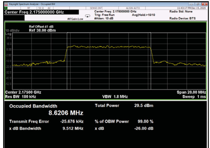
Figure 616: 64QAM 10MHz B.W.; 2175.0MHz, 30kHz - Output
