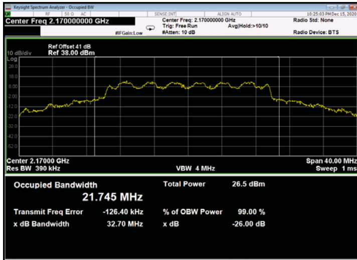
Figure 567: 16QAM 20MHz B.W.; 2170.0MHz, 15kHz - Output
