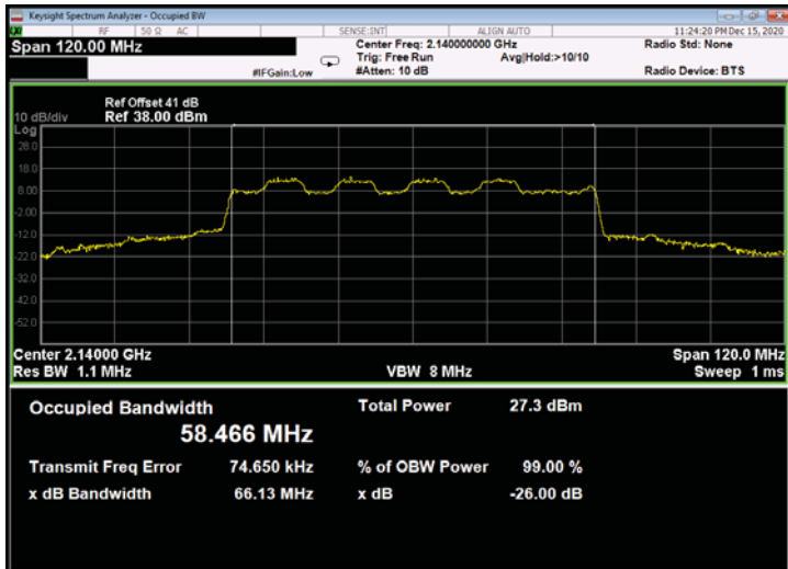
Figure 597: 16QAM 60MHz B.W.; 2140.0MHz, 30kHz - Output
