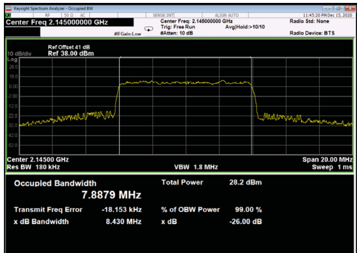
Figure 614: 64QAM 10MHz B.W.; 2145.00MHz, 60kHz - Output
