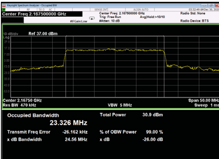
Figure 643: 64QAM 25MHz B.W.; 2167.5MHz, 30kHz - Output
