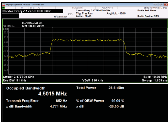
Figure 607: 64QAM 5MHz B.W.; 2177.5MHz, 15kHz - Output
