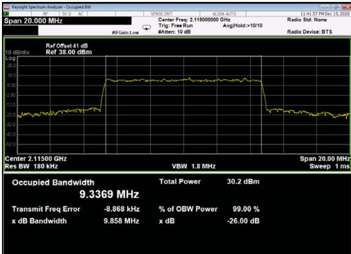
Figure 609: 64QAM 10MHz B.W.; 2115.00MHz, 15kHz - Output
