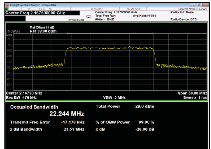
Figure 644: 64QAM 25MHz B.W.; 2167.5MHz, 60kHz - Output
