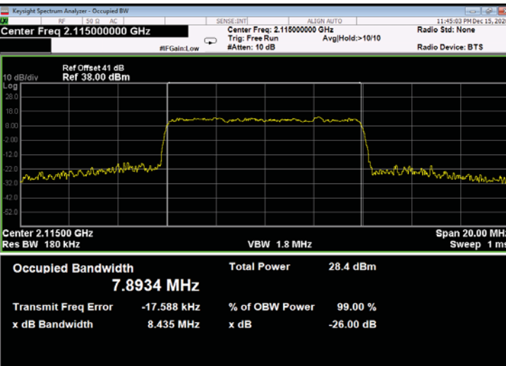
Figure 611: 64QAM 10MHz B.W.; 2115.00MHz, 60kHz - Output
