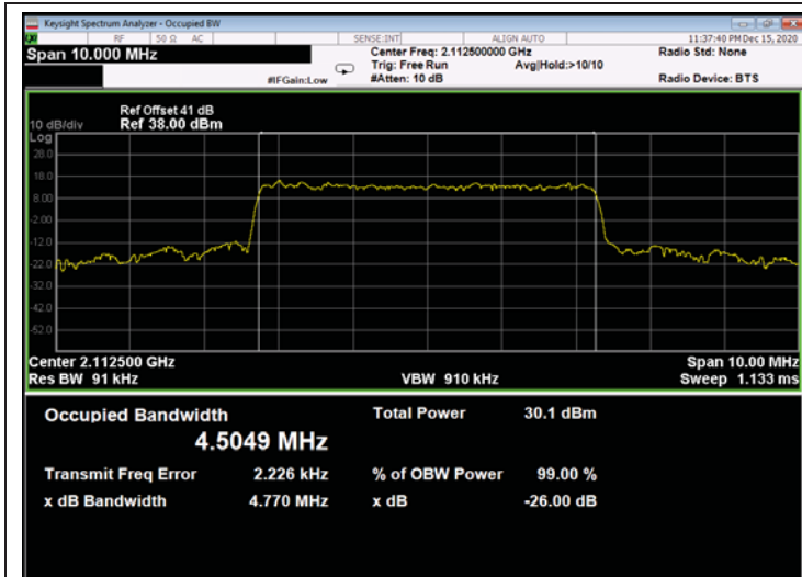
Figure 603: 64QAM 5MHz B.W.; 2112.5MHz, 15kHz - Output
