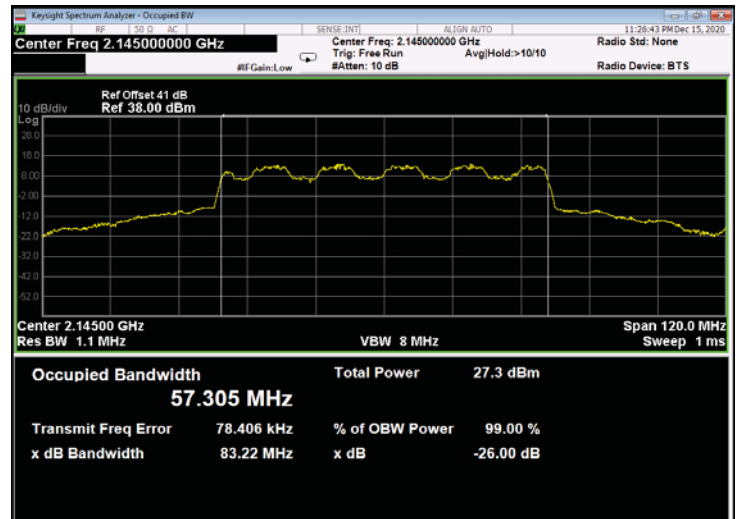
Figure 600: 16QAM 60MHz B.W.; 2145.0MHz, 60kHz - Output
