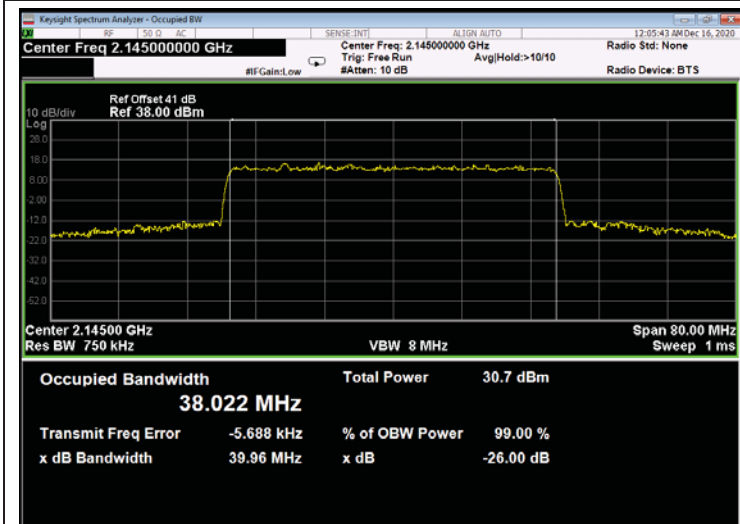
Figure 649: 64QAM 40MHz B.W.; 2145.0MHz, 30kHz - Output
