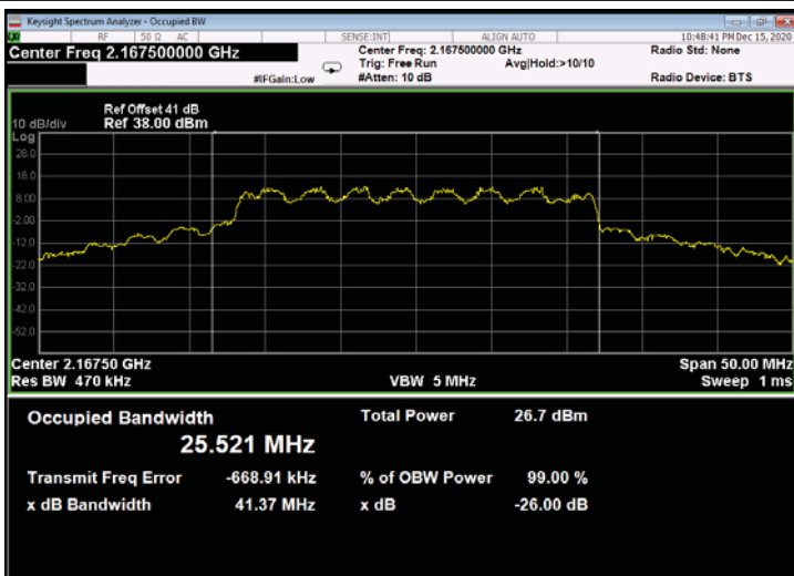
Figure 577: 16QAM 25MHz B.W.; 2167.5MHz, 30kHz - Output
