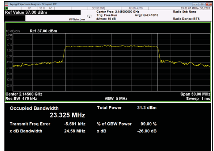
Figure 640: 64QAM 25MHz B.W.; 2145.0MHz, 30kHz - Output
