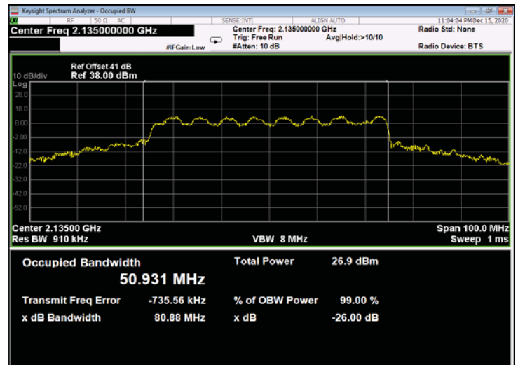
Figure 588: 16QAM 50MHz B.W.; 2135.0MHz, 15kHz - Output
