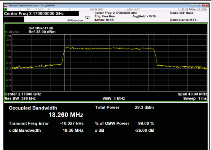
Figure 634: 64QAM 20MHz B.W.; 2170.0MHz, 30kHz - Output
