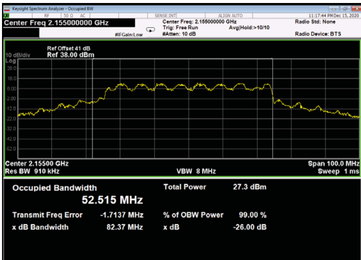
Figure 595: 16QAM 50MHz B.W.; 2155.0MHz, 30kHz - Output
