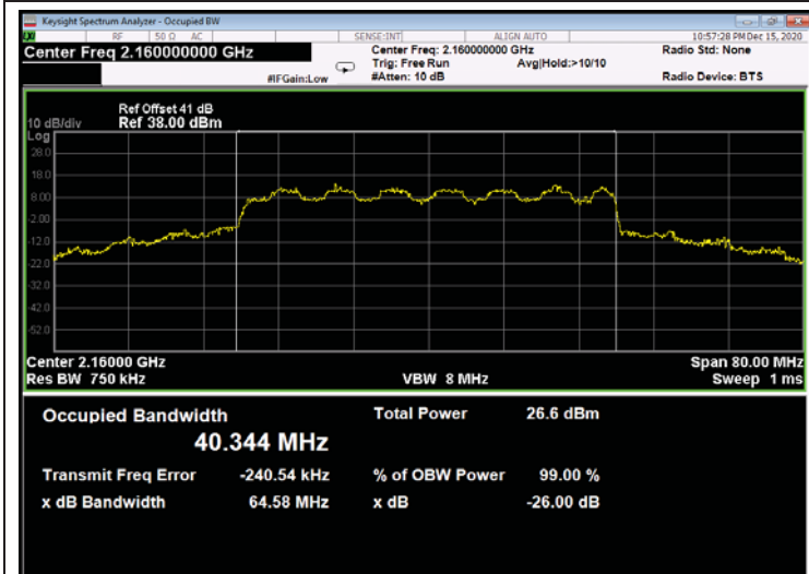
Figure 585: 16QAM 40MHz B.W.; 2160.0MHz, 15kHz - Output
