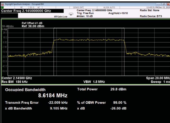
Figure 613: 64QAM 10MHz B.W.; 2145.00MHz, 30kHz - Output
