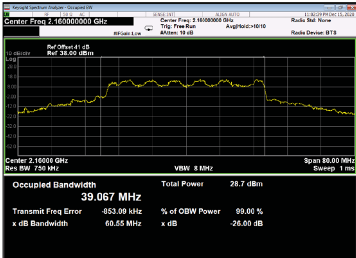
Figure 587: 16QAM 40MHz B.W.; 2160.0MHz, 60kHz - Output
