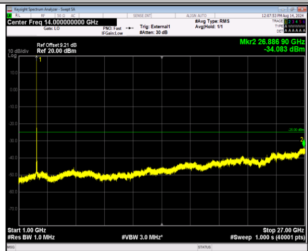
41-41-5MHz-20MHz-QPSK-QPSK-41023-41140-1RB#24-0RB#0-1000~27000MHz-PASS
