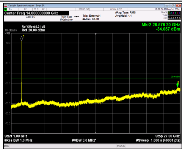
41-41-5MHz-20MHz-QPSK-QPSK-41023-41140-1RB#0-01RB#99-1000~27000MHz-PASS
