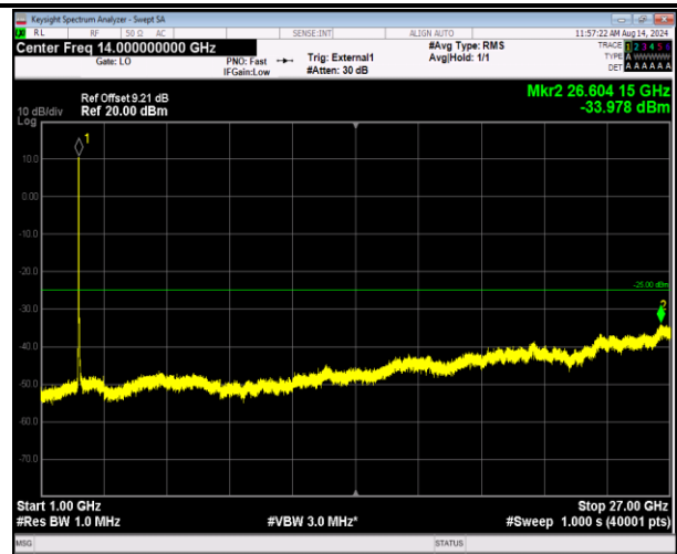
41-41-5MHz-20MHz-QPSK-QPSK-40273-40390-25RB#0-1 00RB#0-1000~27000MHz-PASS
