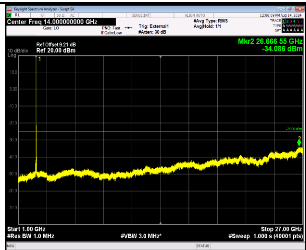
41-41-5MHz-20MHz-QPSK-QPSK-41023-41140-1RB#0-0RB#0-1000~27000MHz-PASS
