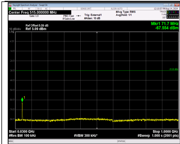
41-41-5MHz-20MHz-QPSK-QPSK-41023-41140-25RB#0 -100RB#0-30~1000MHz-PASS
