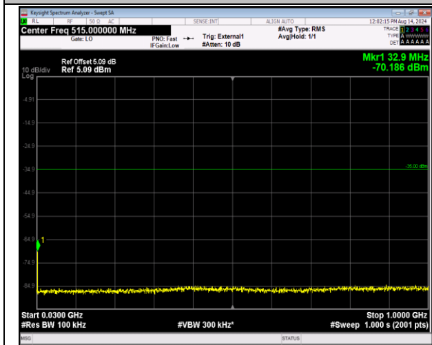
41-41-5MHz-20MHz-QPSK-QPSK-40648-40765-1RB#0-01RB#99-30~1000MHz-PASS
