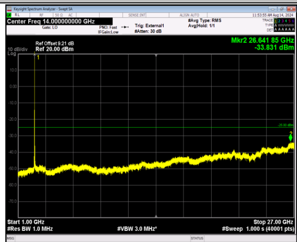
41-41-5MHz-20MHz-QPSK-QPSK-40273-40390-1RB#24-0RB#0-1000~27000MHz-PASS
