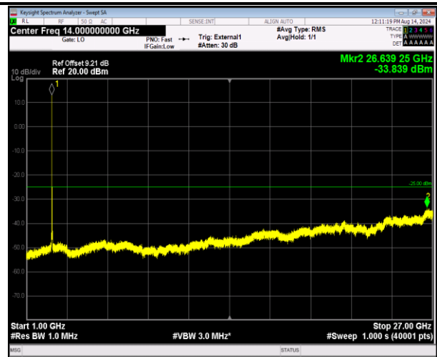
41-41-5MHz-20MHz-QPSK-QPSK-41023-41140-25RB#0-1 00RB#0-1000~27000MHz-PASS
