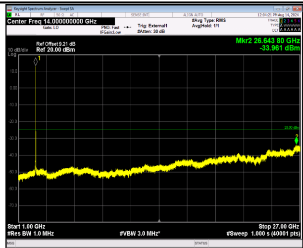
41-41-5MHz-20MHz-QPSK-QPSK-40648-40765-25RB#0-1 00RB#0-1000~27000MHz-PASS
