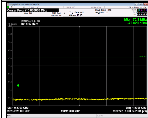
41-41-5MHz-20MHz-QPSK-QPSK-41023-41140-1RB#0-01RB#99-30~1000MHz-PASS
