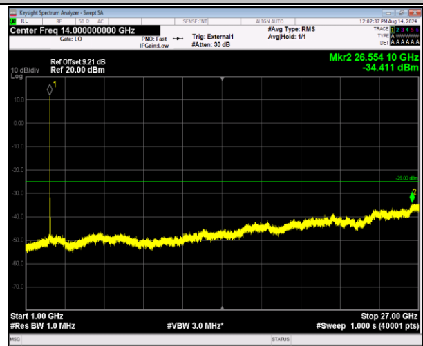
41-41-5MHz-20MHz-QPSK-QPSK-40648-40765-1RB#0-01RB#99-1000~27000MHz-PASS
