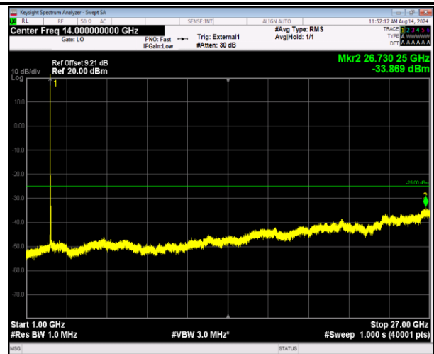
41-41-5MHz-20MHz-QPSK-QPSK-40273-40390-1RB#0-0RB#0-1000~27000MHz-PASS
