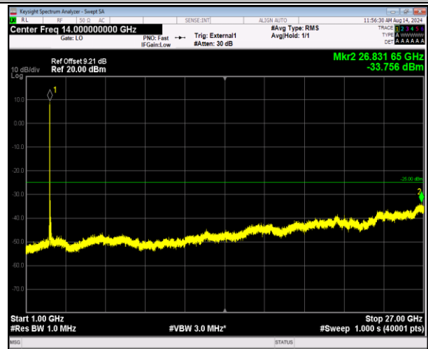
41-41-5MHz-20MHz-16QAM-16QAM-40273-40390-1RB#0- 1RB#99-1000~27000MHz-PASS
