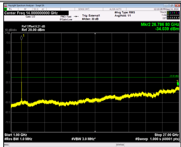
41-41-5MHz-20MHz-16QAM-16QAM-41023-41140-1RB#0- 1RB#99-1000~27000MHz-PASS
