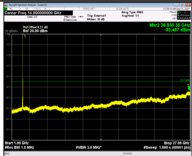
41-41-5MHz-20MHz-QPSK-QPSK-40648-40765-1RB#0-0RB#0-1000~27000MHz-PASS
