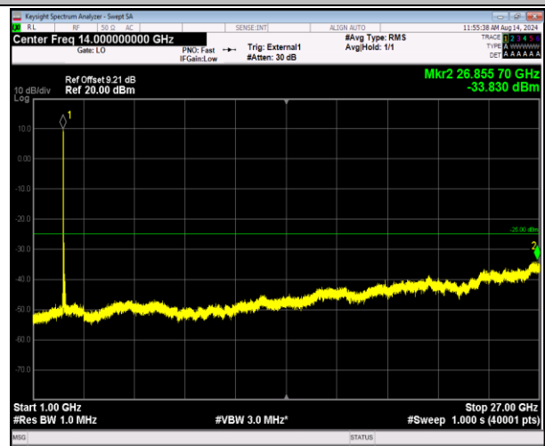
41-41-5MHz-20MHz-QPSK-QPSK-40273-40390-1RB#0-01RB#99-1000~27000MHz-PASS
