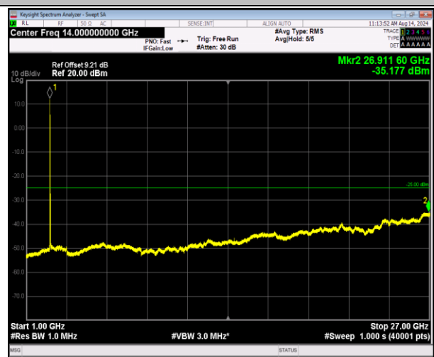
7-7-20MHz-20MHz-QPSK-QPSK-21152-21350-1RB#0-1RB #99-1000~27000MHz-PASS
