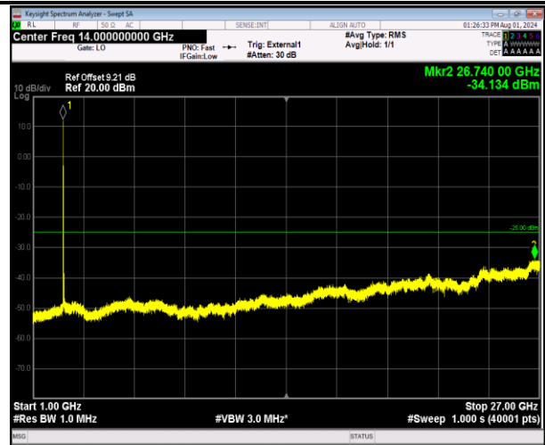
41-41-5MHz-20MHz-64QAM-64QAM-40273-40390-1RB#0- 1RB#99-1000~27000MHz-PASS
