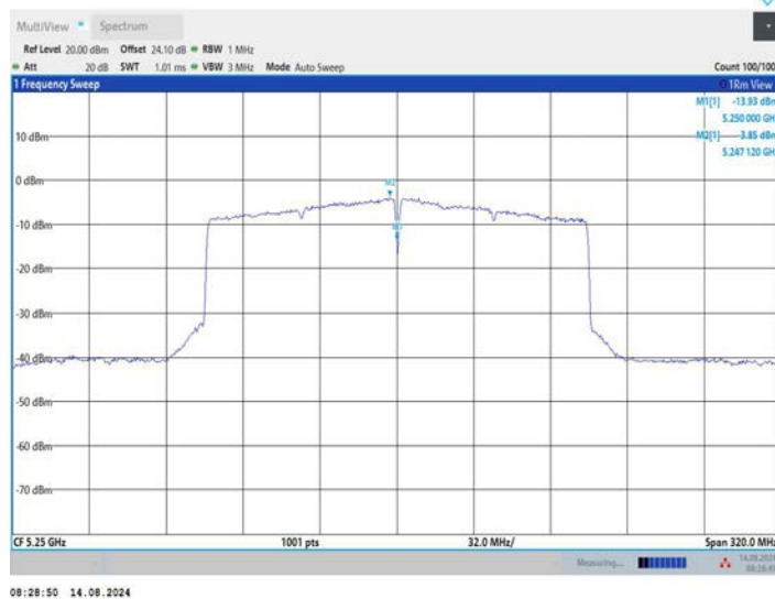
11BE160MIMO_Ant2_5250_UNII-1
