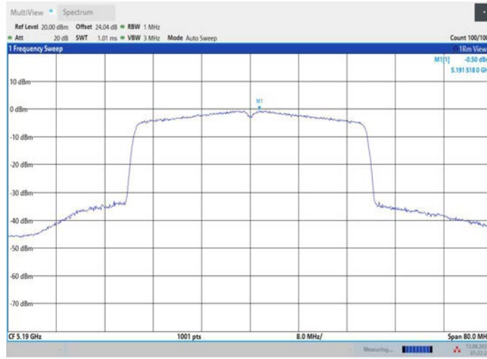
11BE40MIMO_Ant3_5190
