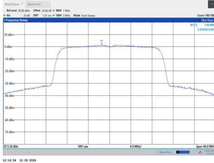
11BE20MIMO_Ant2_5320
