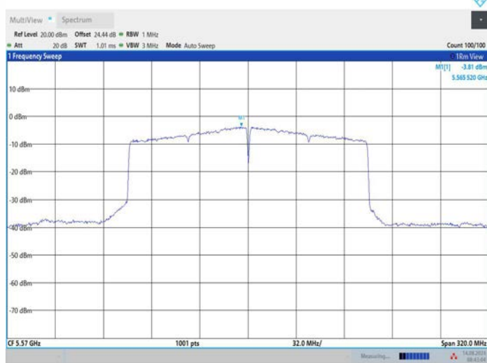
11BE160MIMO_Ant3_5570
