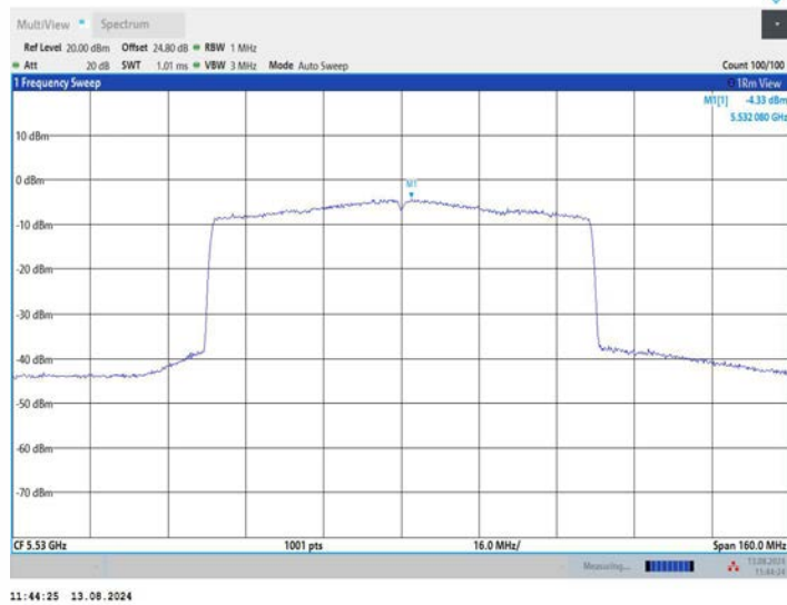
11BE80MIMO_Ant3_5530
