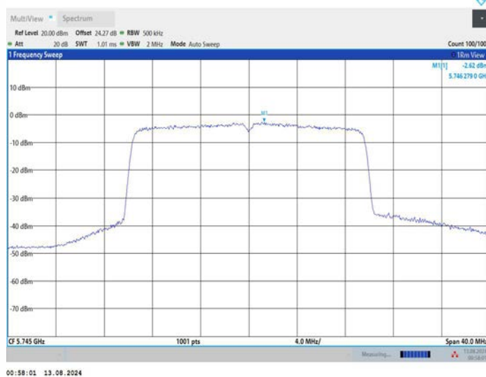
11BE20MIMO_Ant3_5745
