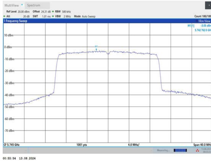
11BE20MIMO_Ant2_5745
