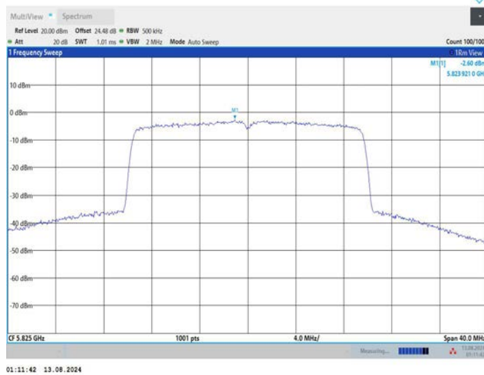
11BE20MIMO_Ant3_5825
