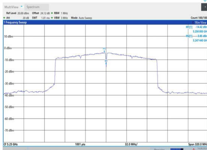
11BE160MIMO_Ant1_5250_UNII-2A
