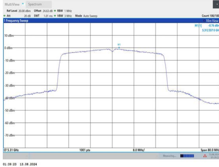
11BE40MIMO_Ant2_5310
