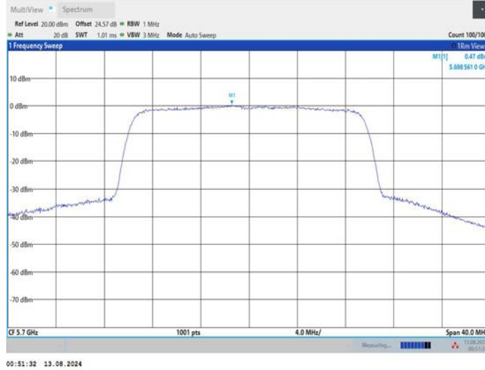
11BE20MIMO_Ant3_5700
