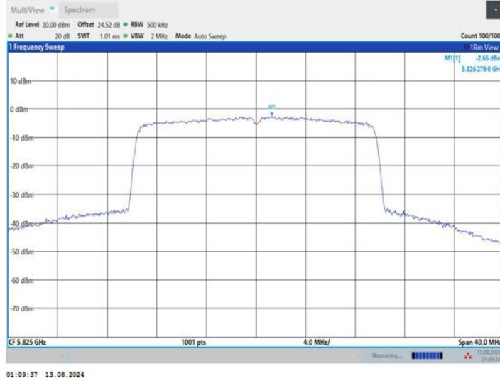
11BE20MIMO_Ant2_5825
