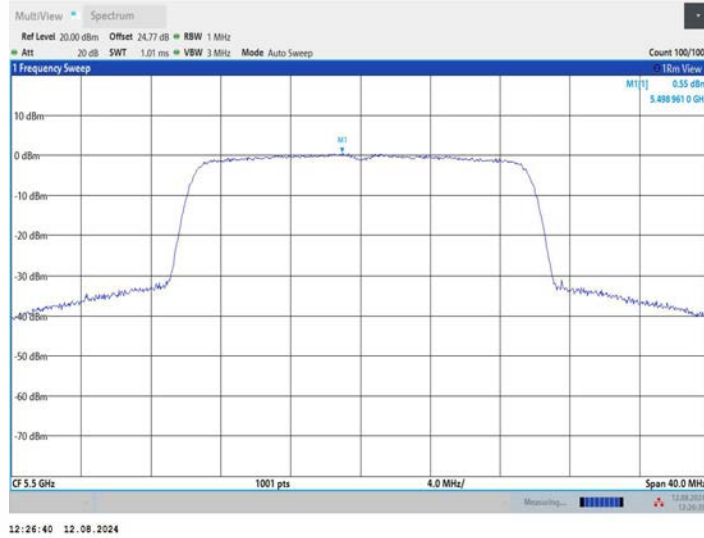
11BE20MIMO_Ant3_5500
