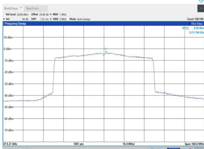
11BE80MIMO_Ant3_5210
