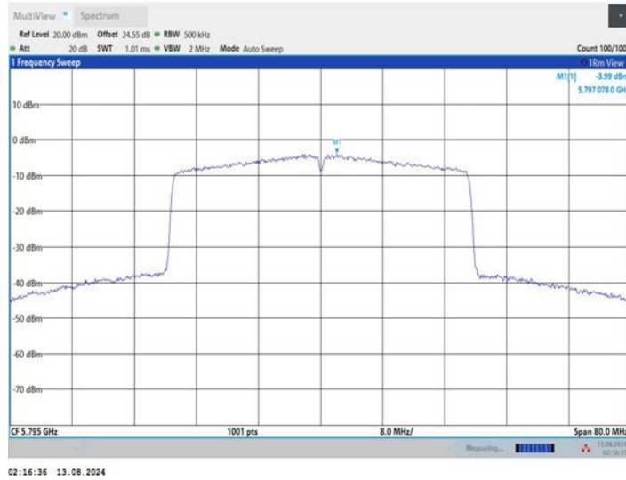
11BE40MIMO_Ant3_5795
