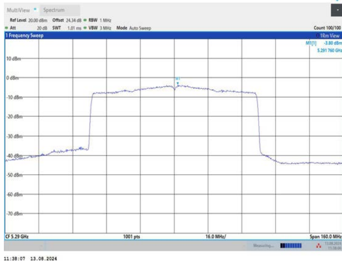
11BE80MIMO_Ant3_5290
