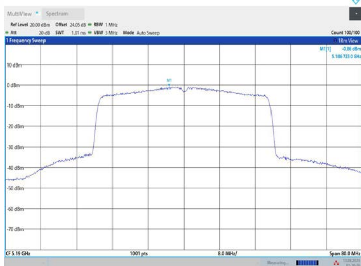
11BE40MIMO_Ant2_5190
