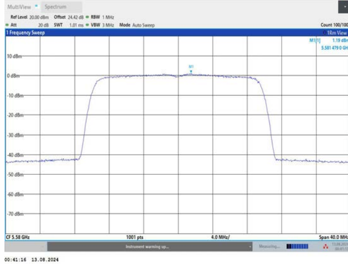
11BE20MIMO_Ant2_5580
