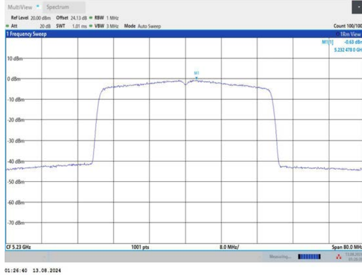
11BE40MIMO_Ant2_5230
