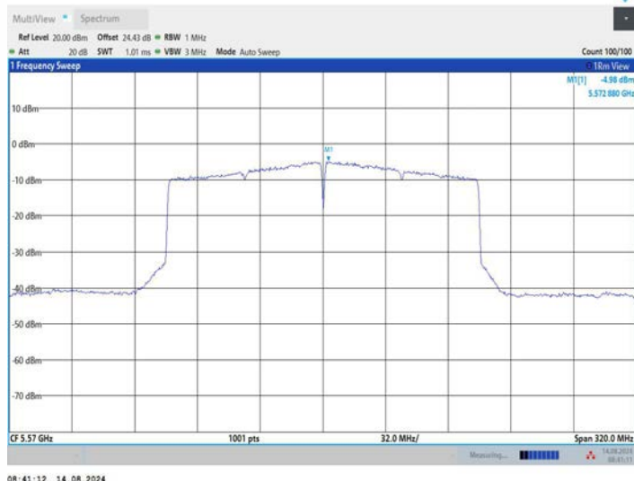
11BE160MIMO_Ant3_5570
