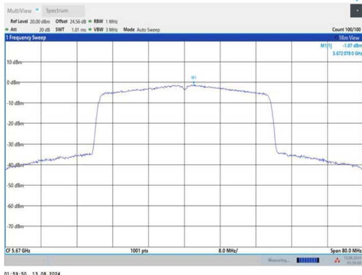
11BE40MIMO_Ant3_5670
