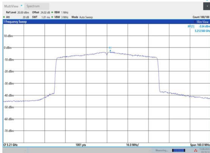
11BE80MIMO_Ant2_5210
