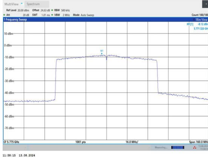
11BE80MIMO_Ant2_5775
