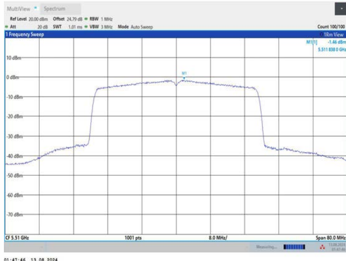
11BE40MIMO_Ant3_5510
