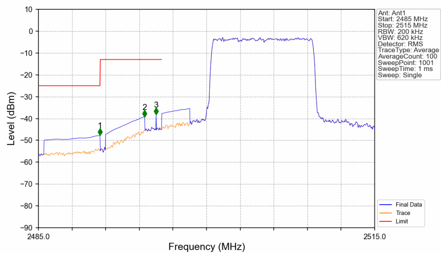
Band7_10MHz_QPSK_LCH_2505MHz_RB_50_0_NTNV
