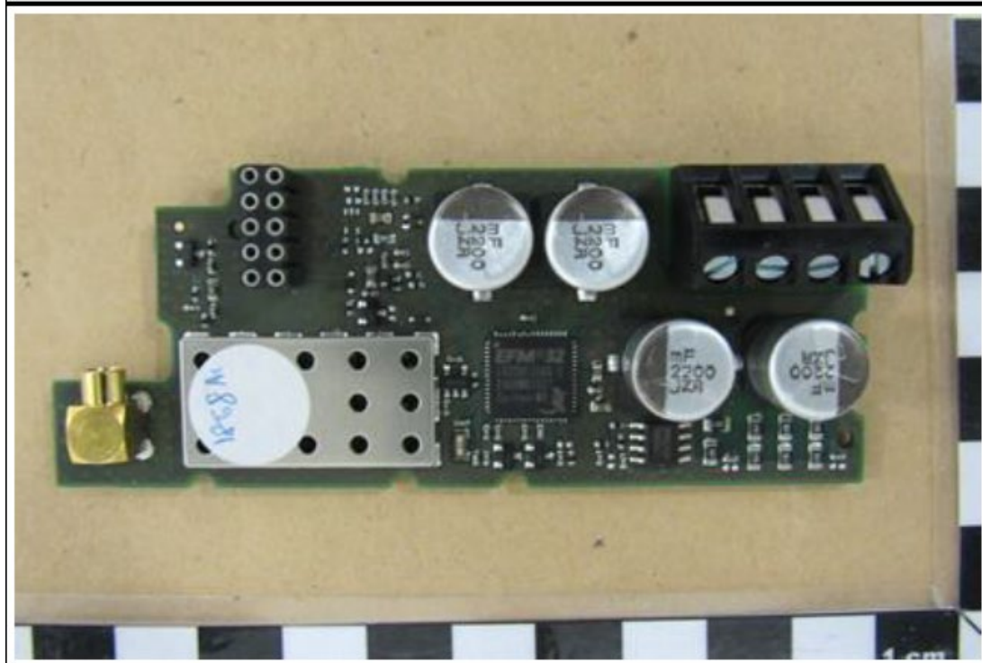
EUT TOP SIDE
