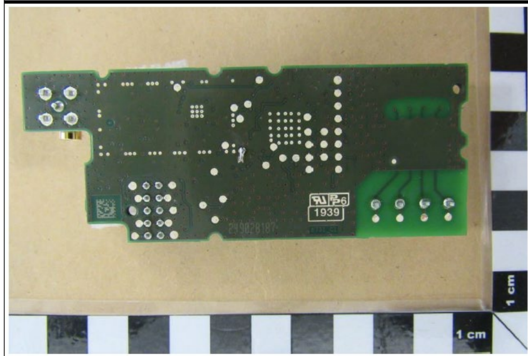
5550 1868 A3 (radio module bottom view)
