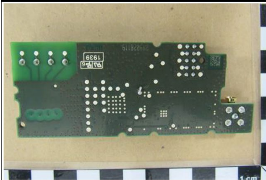
EUT BOTTOM SIDE
