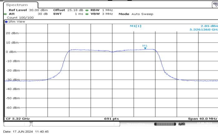
11A-CDD_Ant3_5320
