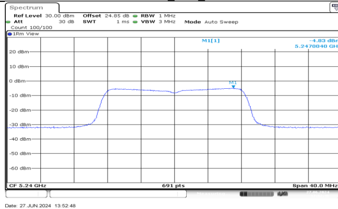
11A-CDD_Ant1_5240
