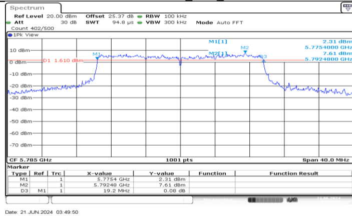
11AX20MIMO_Ant4_5785
