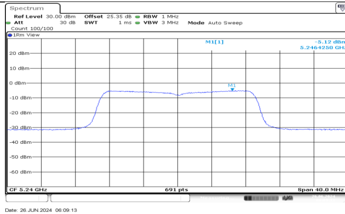
11AC20MIMO_Ant2_5240
