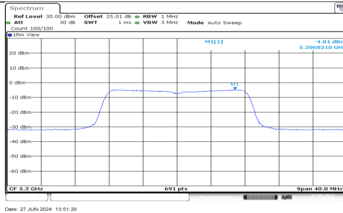
11A-CDD_Ant3_5200
