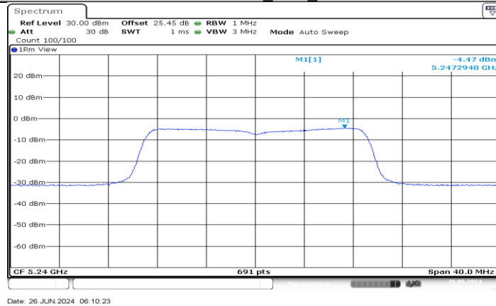
11AC20MIMO_Ant4_5240
