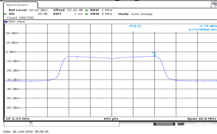
11AC20MIMO_Ant3_5240
