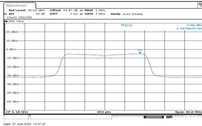
11A-CDD Ant1 5180
