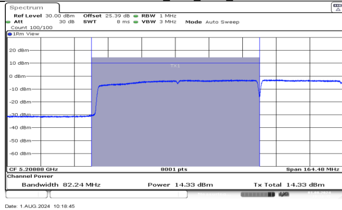
11AX160MIMO_Ant3_5250_UNII-1
