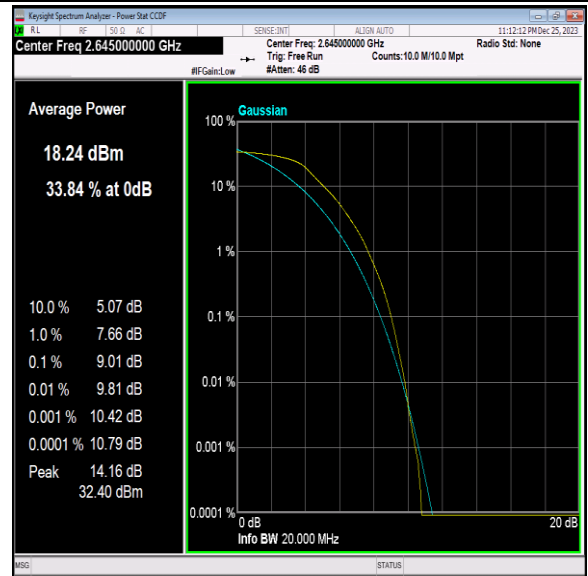
41(2535-2655)-20MHz-QPSK-41140-100RB#0-PASS
