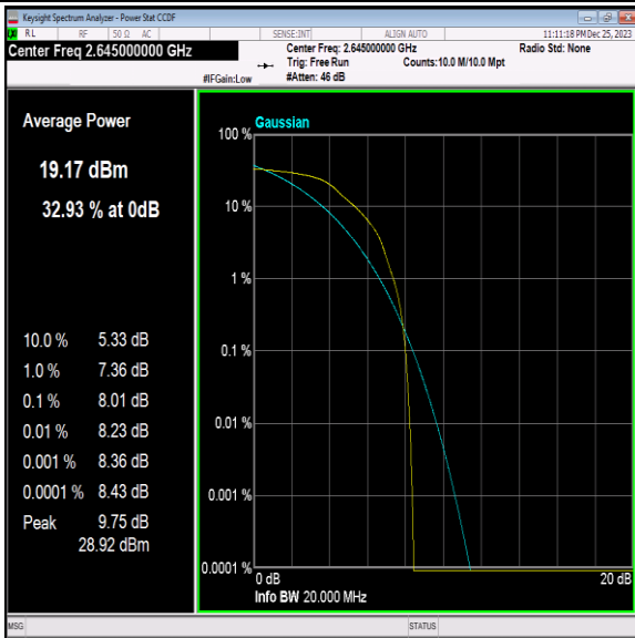
41(2535-2655)-20MHz-QPSK-41140-1RB#0-PASS
