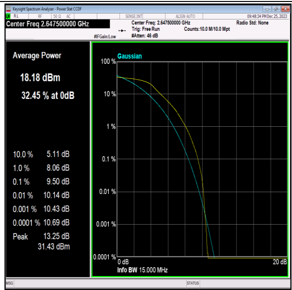
41(2535-2655)-15MHz-QPSK-41165-75RB#0-PASS
