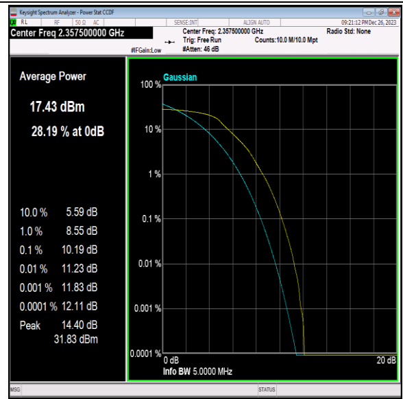
40(2350-2360)-5MHz-QPSK-39225-25RB#0-PASS
