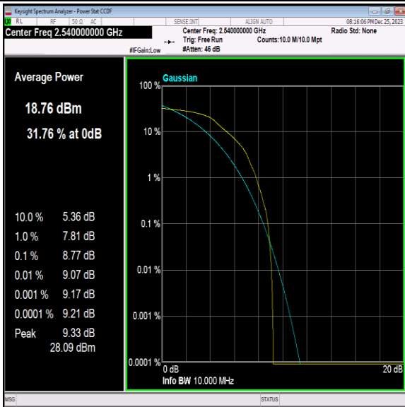
41(2535-2655)-10MHz-QPSK-40090-1RB#0-PASS
