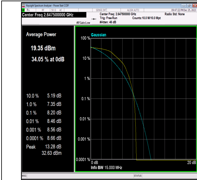
41(2535-2655)-15MHz-QPSK-41165-1RB#0-PASS
