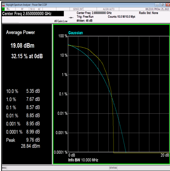
41(2535-2655)-10MHz-64QAM-41190-1RB#0-PASS
