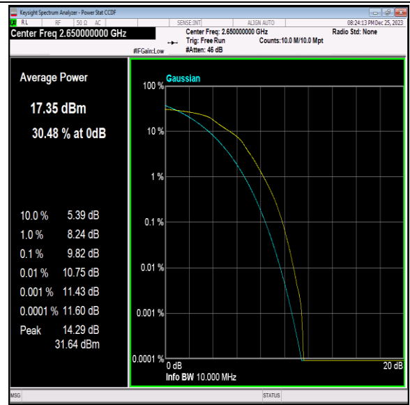
41(2535-2655)-10MHz-16QAM-41190-50RB#0-PASS
