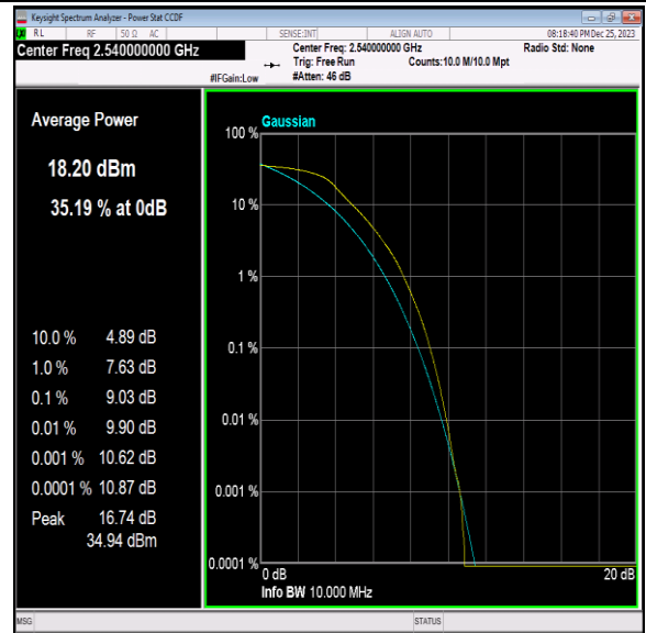
41(2535-2655)-10MHz-64QAM-40090-50RB#0-PASS
