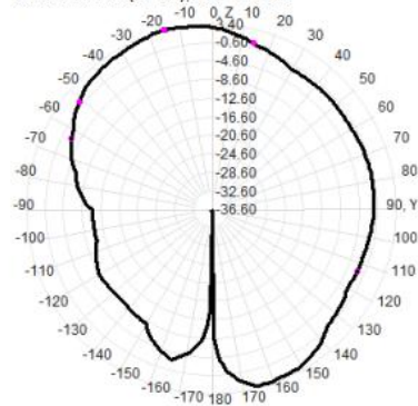
2400.0MHz Total(E2-YZ), Max= 3.40dBi
