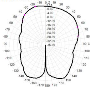
2440.0MHz Total(E1-XZ), Max= 2.91dBi
