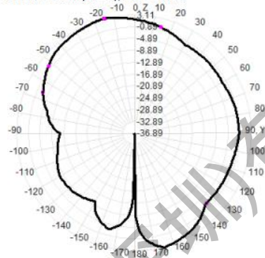
2440.0MHz Total(E2-YZ), Max= 3.11dBi
