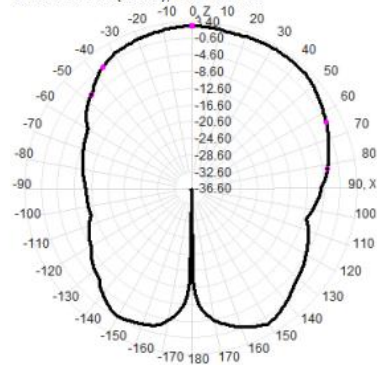
2400.0MHz Total(E1-XZ), Max= 2.40dBi
