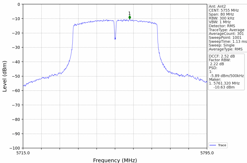
802.11ac(VHT40)_LCH_5755MHz_MIMO_NTNV
