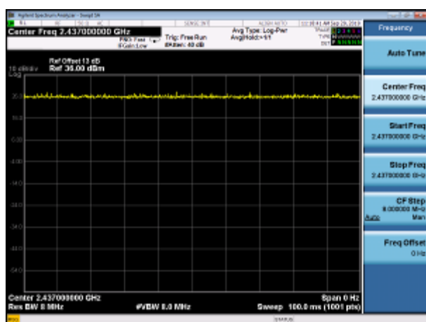
802.11n(20MHz)(2437MHz)
