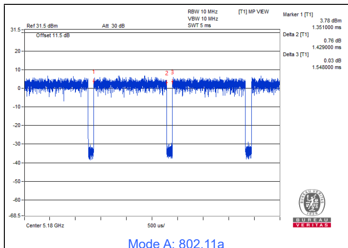
Mode A: 802.11a
