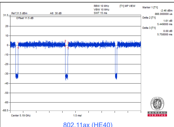
802.11ax (HE40)
