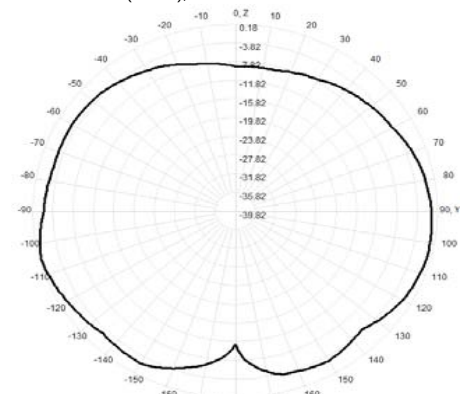
920.0MHz Total(E2-YZ), Max= -0.17dBi
