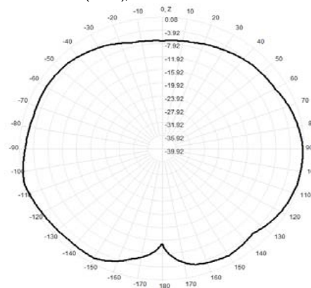
890.0MHz Total(E2-YZ), Max= 0.08dBi
