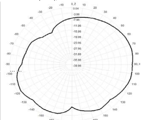
930.0MHz Total(E1-XZ), Max= 0.04dBi
