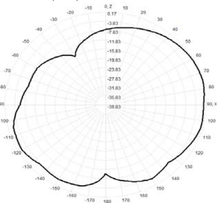
910.0MHz Total(E1-XZ), Max= 0.17dBi
