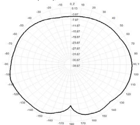
880.0MHz Total(E2-YZ), Max= 0.13dBi
