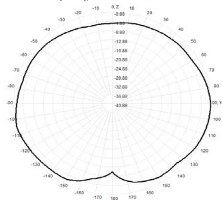
860.0MHz Total(E2-YZ), Max= -0.90dBi
