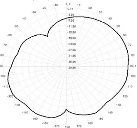
900.0MHz Total(E1-XZ), Max= 0.14dBi
