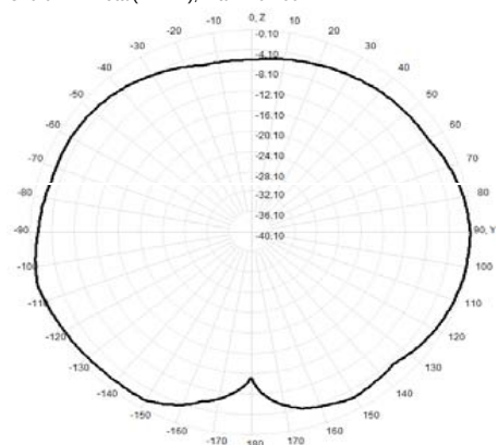
870.0MHz Total(E2-YZ), Max= -0.10dBi
