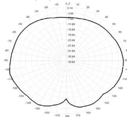
900.0MHz Total(E2-YZ), Max= 0.03dBi
