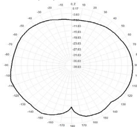
910.0MHz Total(E2-YZ), Max= -0.04dBi
