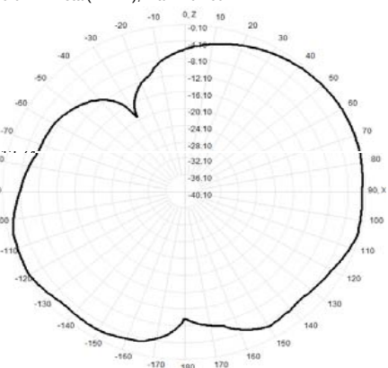
870.0MHz Total(E1-XZ), Max= -0.20dBi
