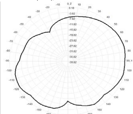
920.0MHz Total(E1-XZ), Max= 0.18dBi
