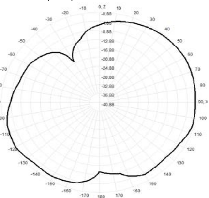
860.0MHz Total(E1-XZ), Max= -0.88dBi
