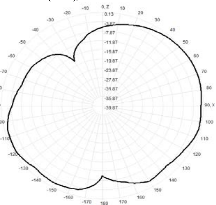
880.0MHz Total(E1-XZ), Max= -0.08dBi
