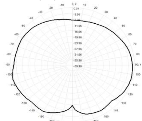
930.0MHz Total(E2-YZ), Max= -0.47dBi
