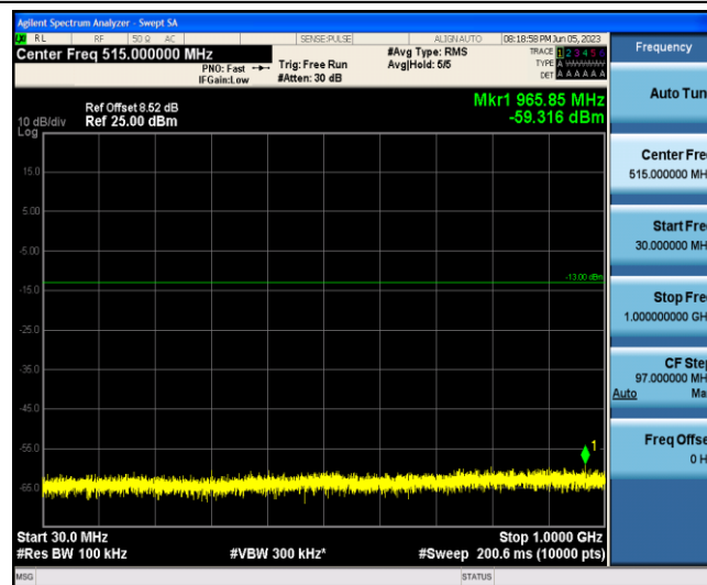
Band2-10MHz-QPSK-19150-1-0-Low-30-1000--59.32-PASS
