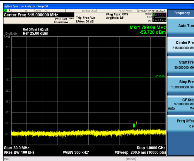
Band2-5MHz-QPSK-19175-1-0-Low-30-1000--59.72-PASS
