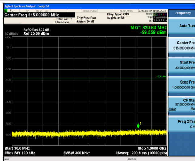
Band2-5MHz-16QAM-18900-1-0-Low-30-1000--59.56-PASS
