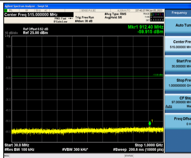
Band2-3MHz-QPSK-19185-1-0-Low-30-1000--59.92-PASS
