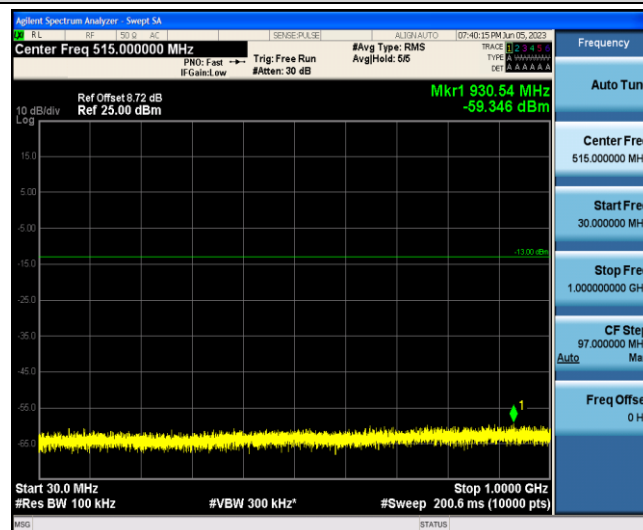
Band2-3MHz-16QAM-18900-1-0-Low-30-1000--59.35-PASS
