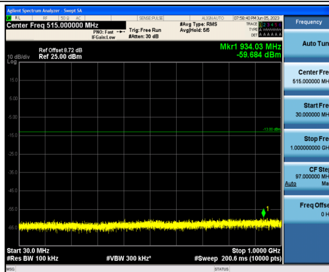
Band2-5MHz-QPSK-18900-1-0-Low-30-1000--59.68-PASS
