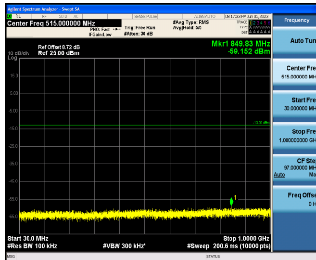
Band2-10MHz-QPSK-18650-1-0-Low-30-1000--59.15-PASS
