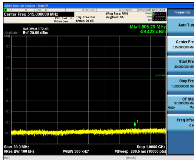
Band2-5MHz-QPSK-18625-1-0-Low-30-1000--59.42-PASS
