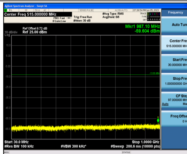
Band2-3MHz-QPSK-18900-1-0-Low-30-1000--59.6-PASS
