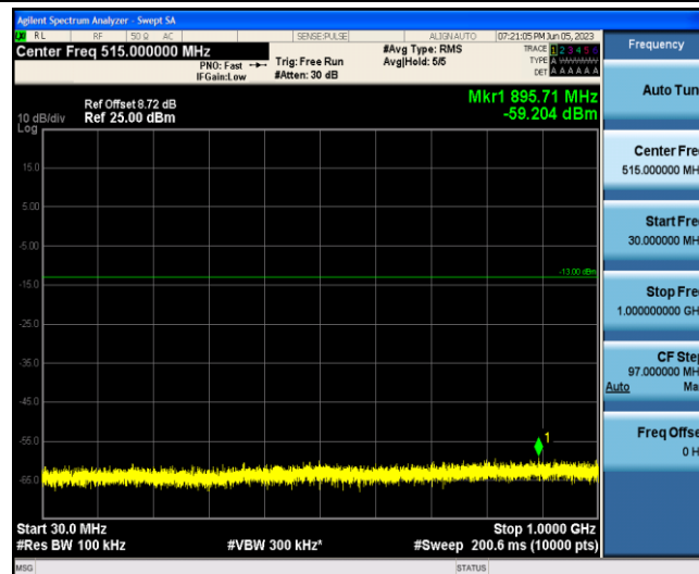
Band2-1.4MHz-QPSK-18900-1-0-Low-30-1000--59.2-PASS
