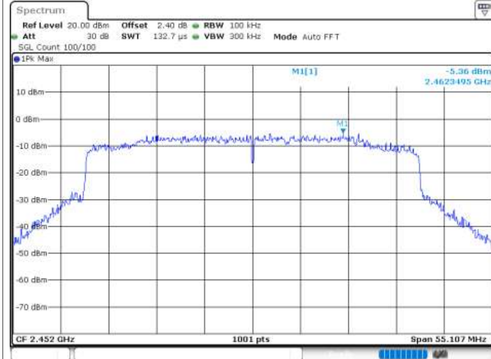
PSD NVNT ax40 2452MHz Ant1
